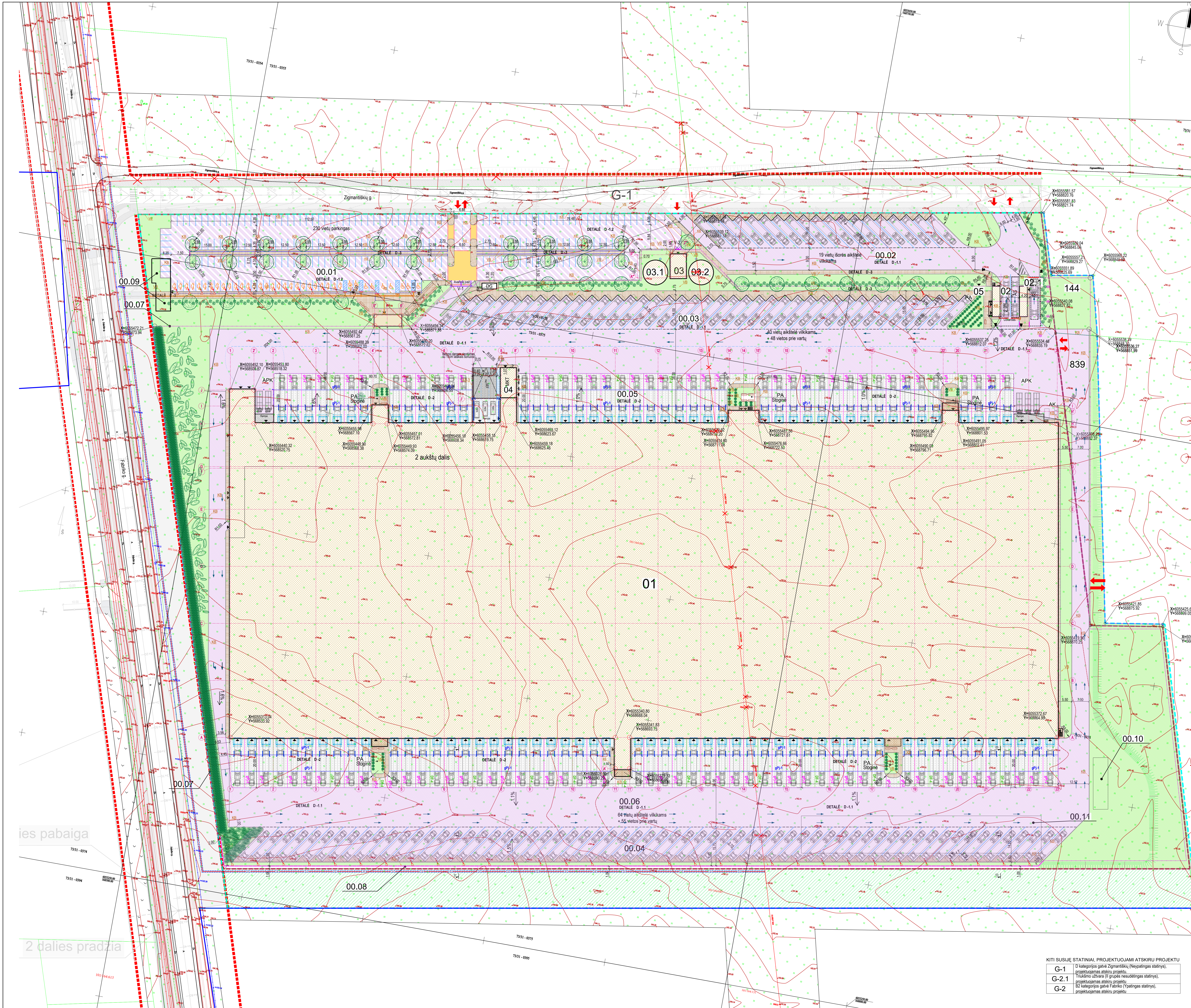
SITUACIJOS SCHEMA M 1:10 000
