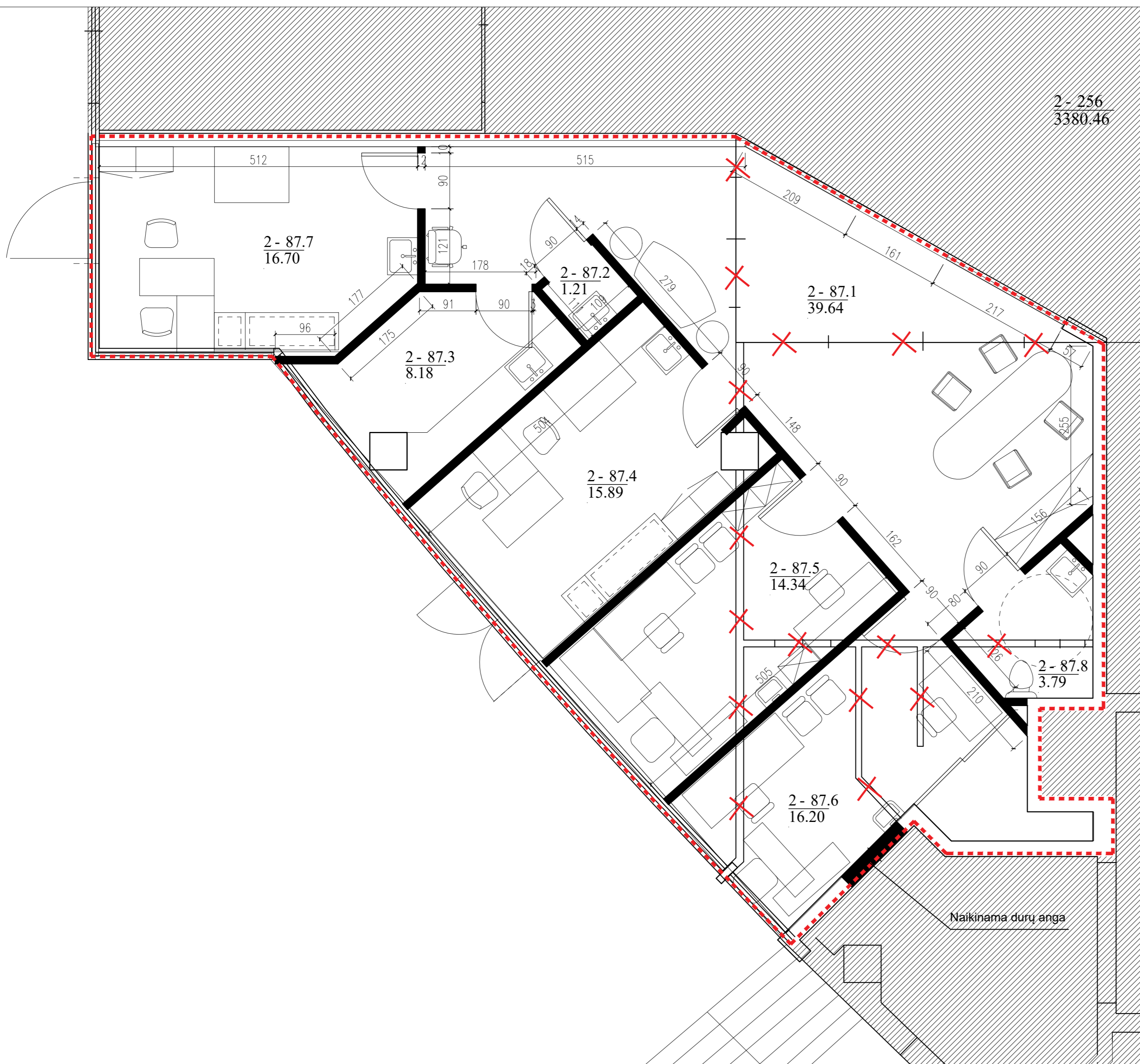
Projektuojamų patalpų planas. M1:50
