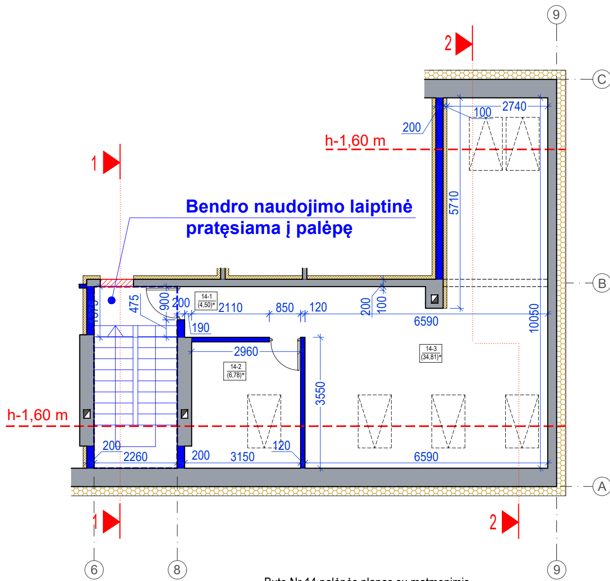
Buto Nr.14 palėpės planas su matmenimis.
