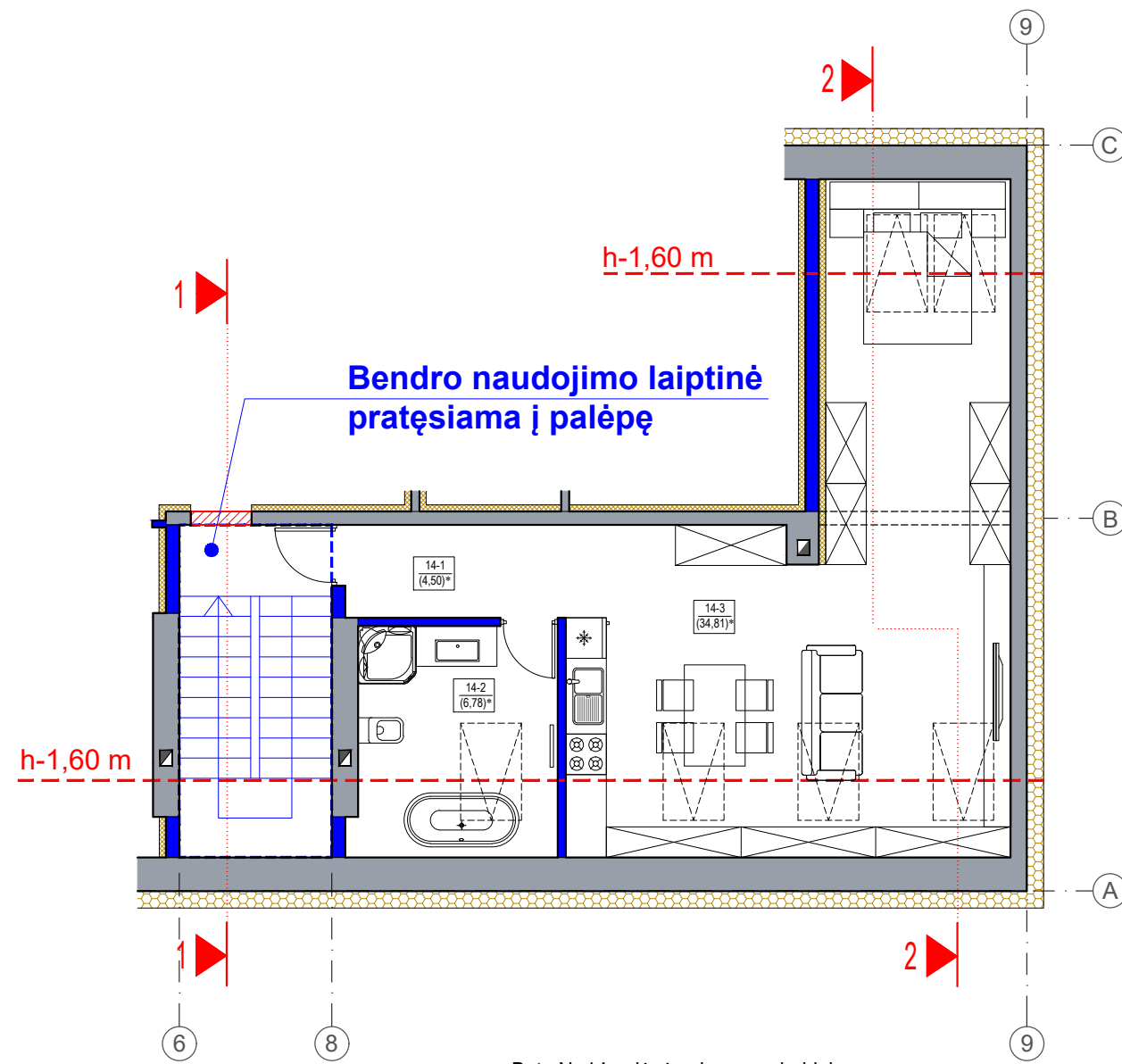
Buto Nr.14 palėpės planas su baldais.
