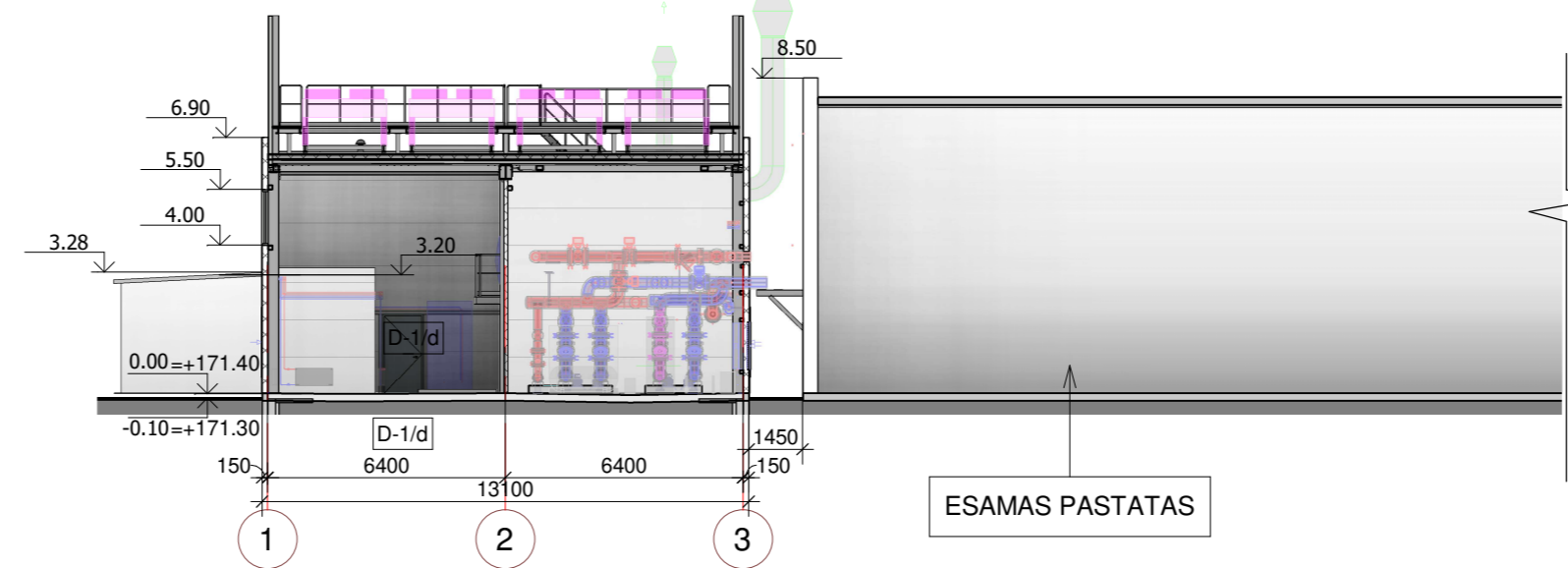
PJŪVIS 2-2
