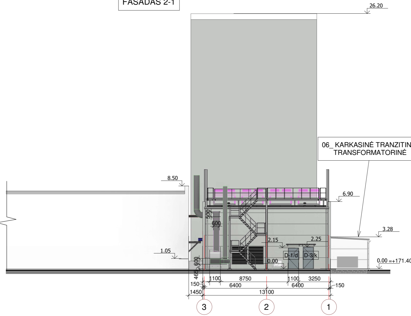
FASADAS 2-1
