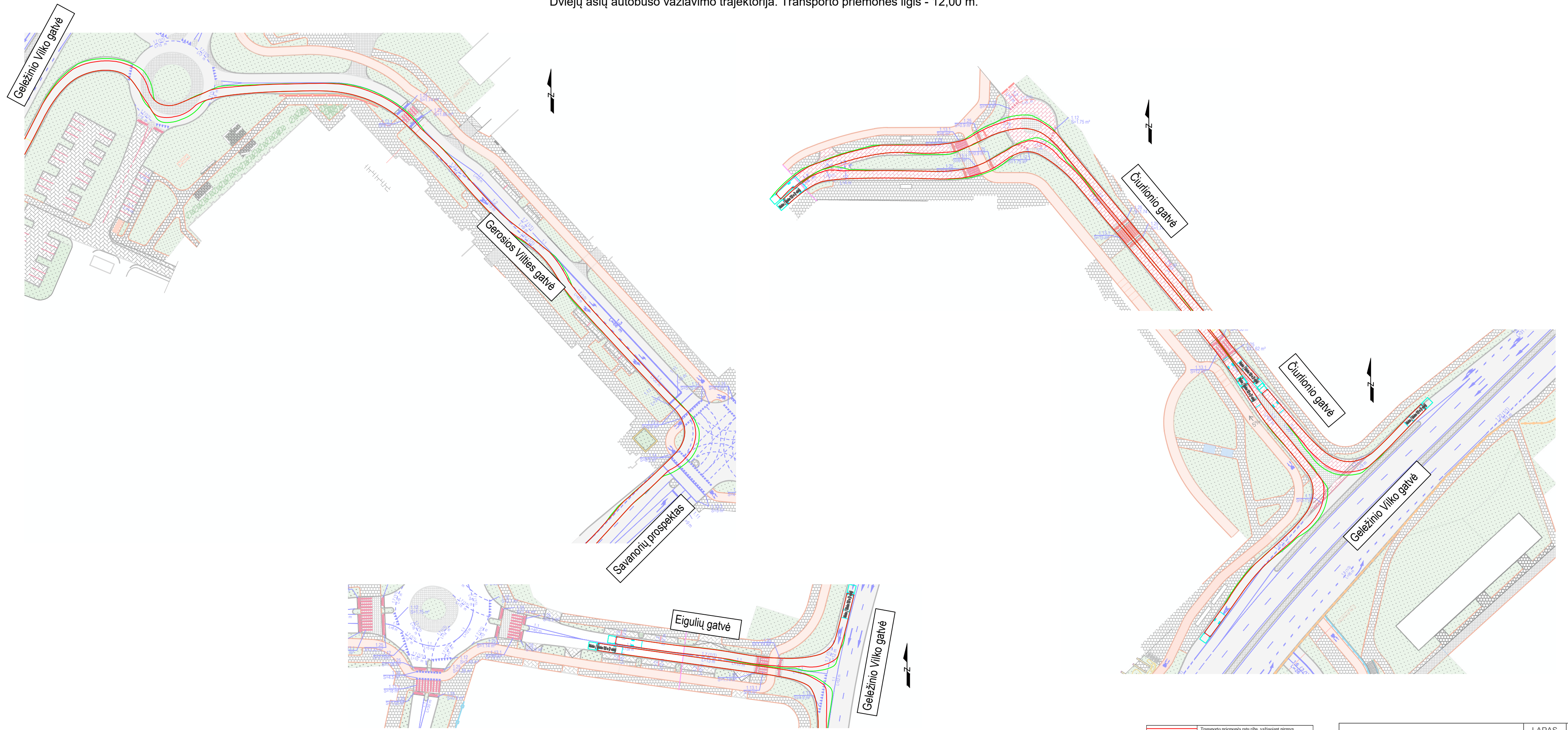
Dviejų ašių autobuso važiavimo trajektorija. Transporto priemonės ilgis - 12,00 m.
