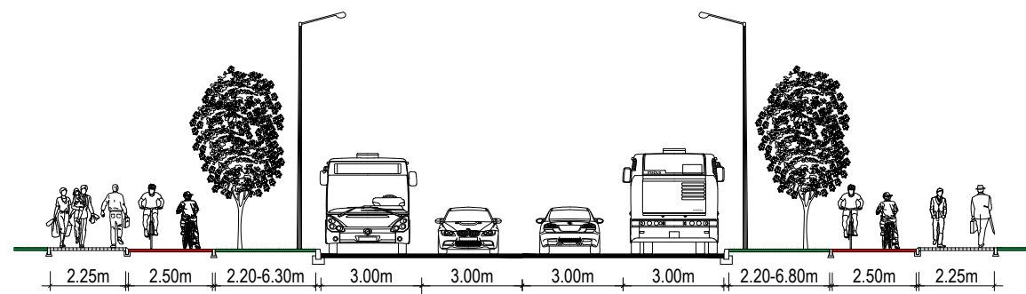
Pjūvis 1 - 1 Pavilnionių g.
