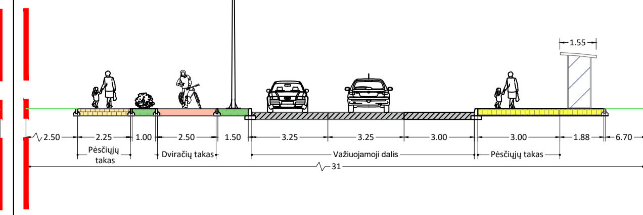
Jungiamojo kelio skersinis pjūvis 5-5
