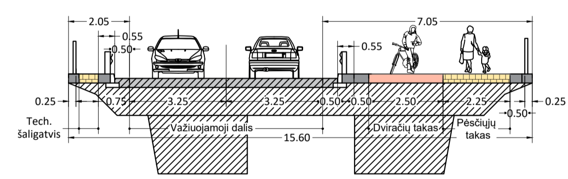
Minsko pl. skersinis pjūvis 2-2
