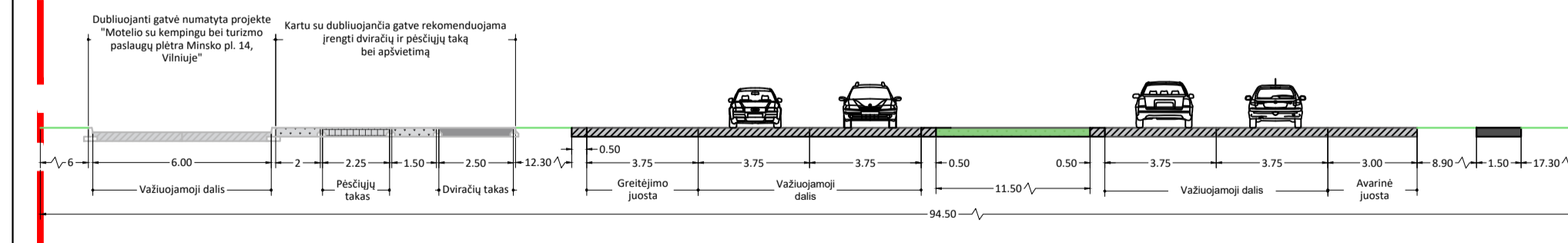
Minsko pl. skersinis pjūvis 2-2
