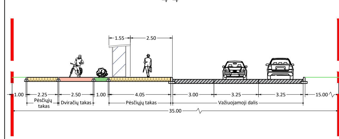
Gurių g. skersinis pjūvis 4-4
