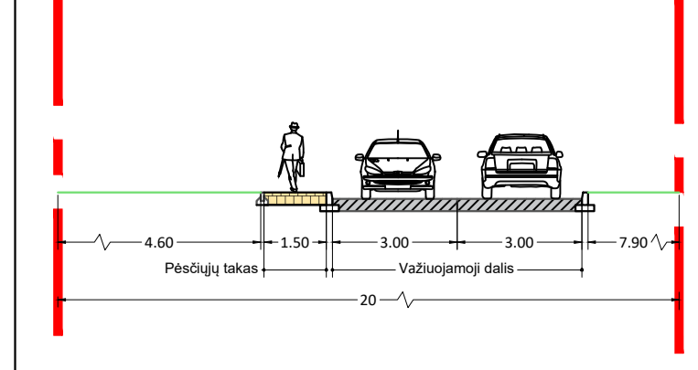
Ušos g. skersinis pjūvis (esamas) 3-3
