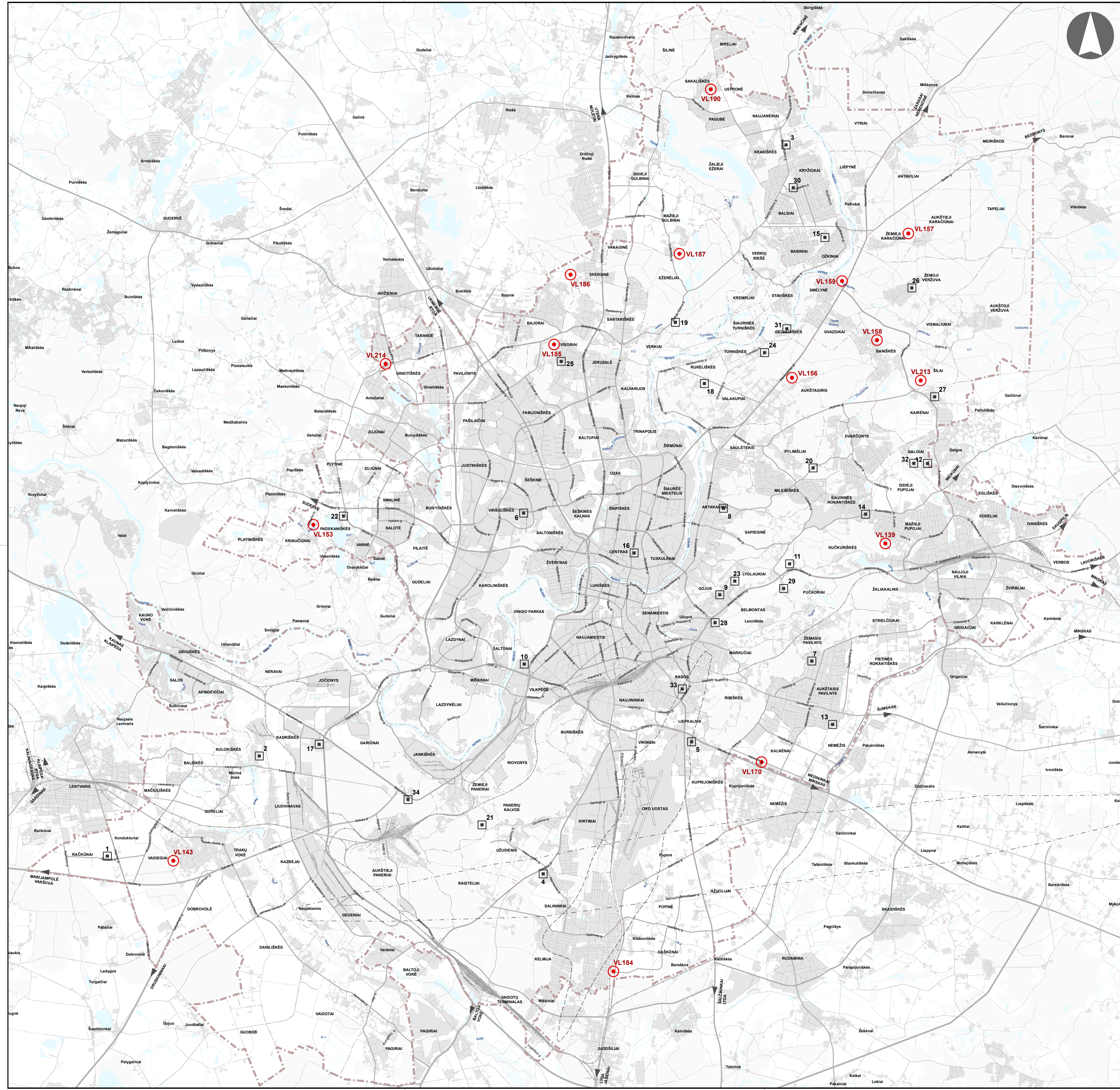
Schema parengta vadovaujantis Vilniaus miesto savivaldybės teritorijos skaitmeninio radijo ryšio tinklo bazinių stočių išdėstymo schema, patvirtinta Vilniaus miesto savivaldybės tarybos 2008-04-23 sprendimu Nr. 1-449
