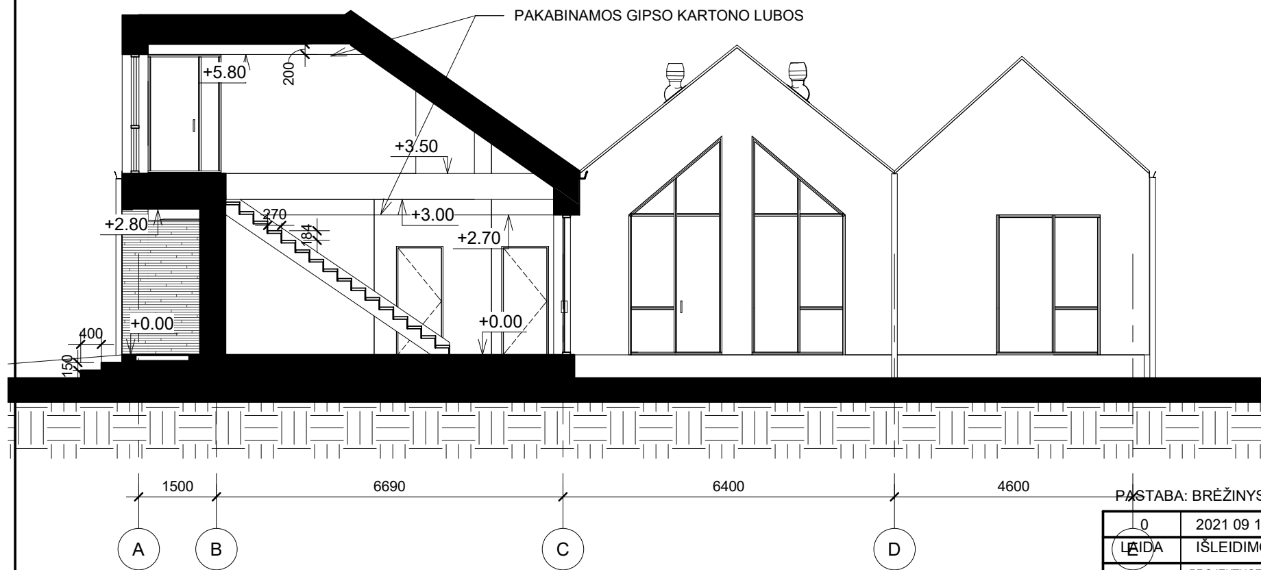
PJŪVIS 3-3
