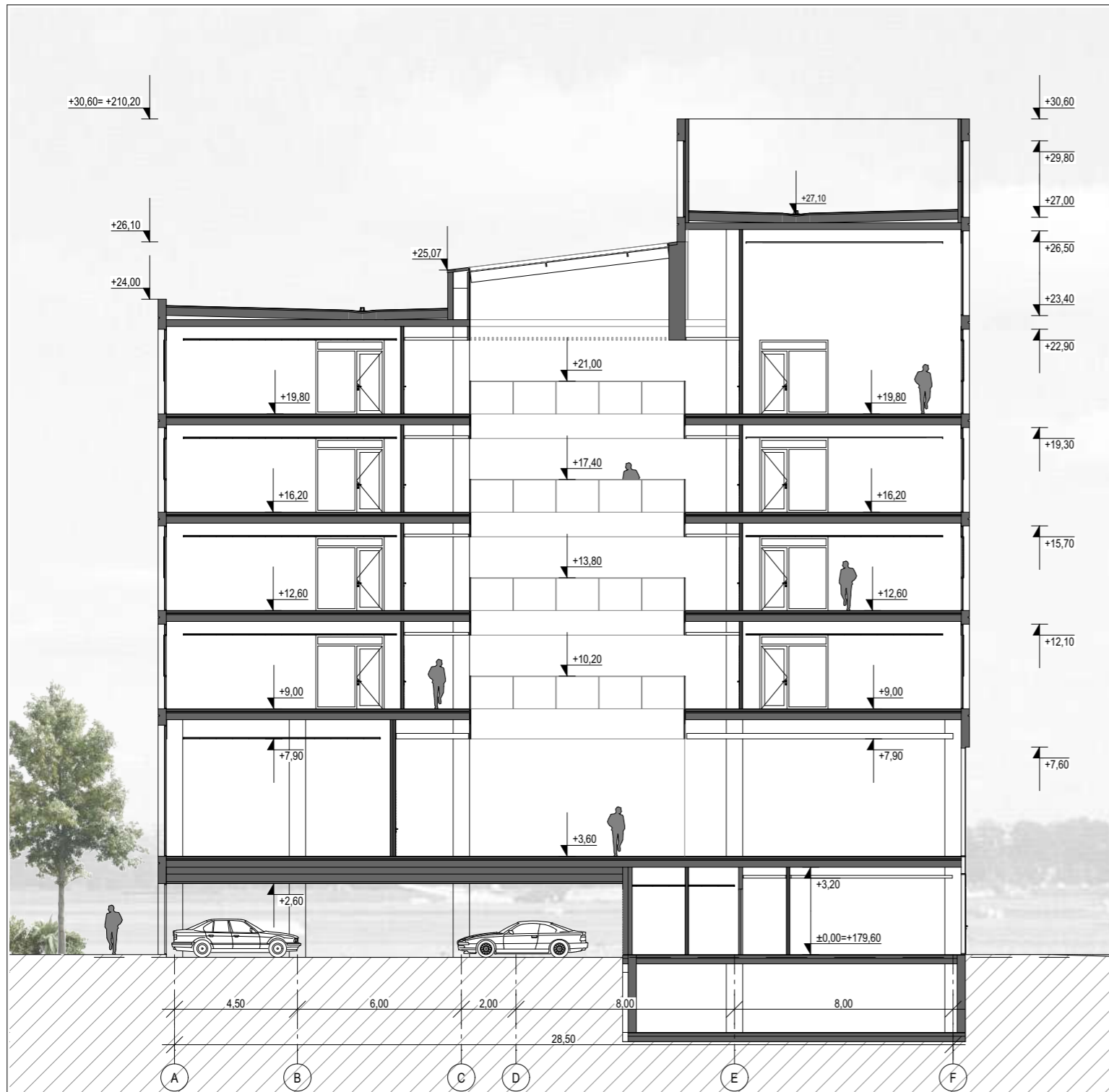
1-1 PJŪVIS
