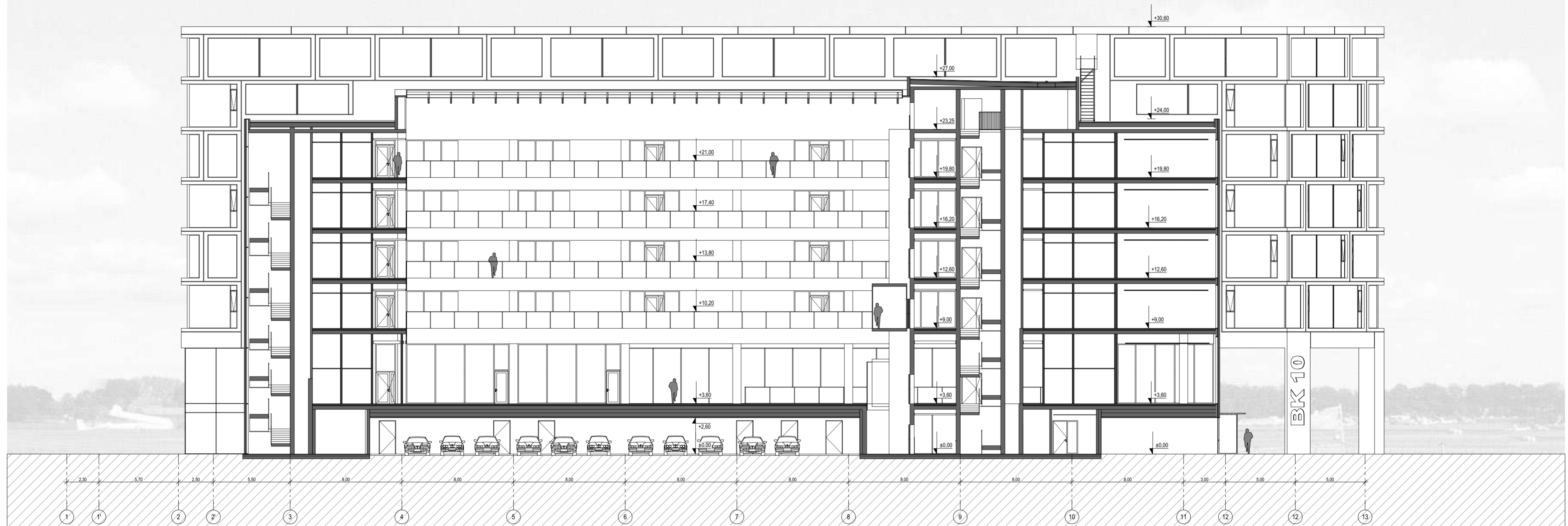
5-5 PJŪVIS
