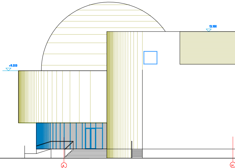
FASADAS A-H
