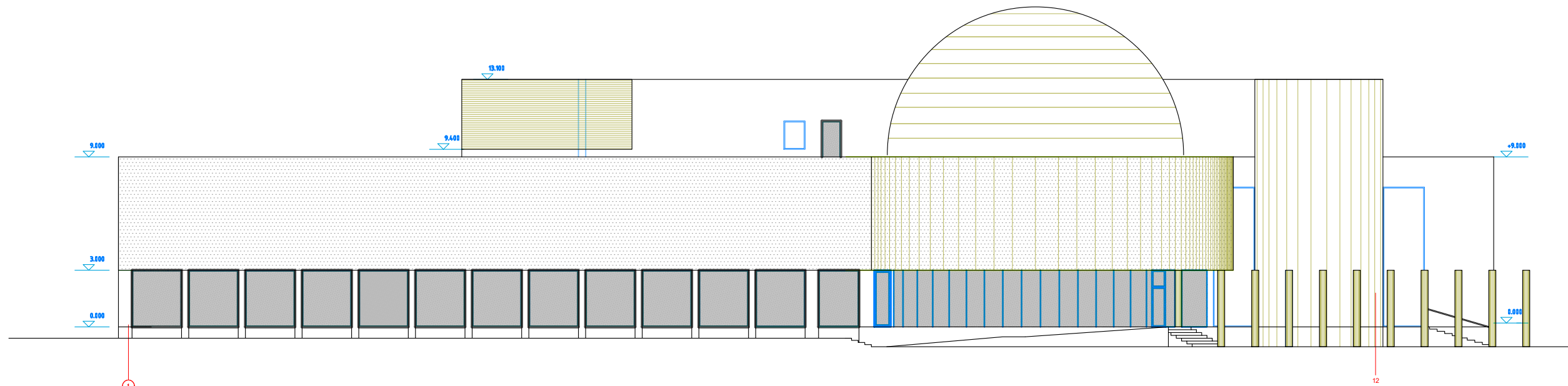
FASADAS 1-12
