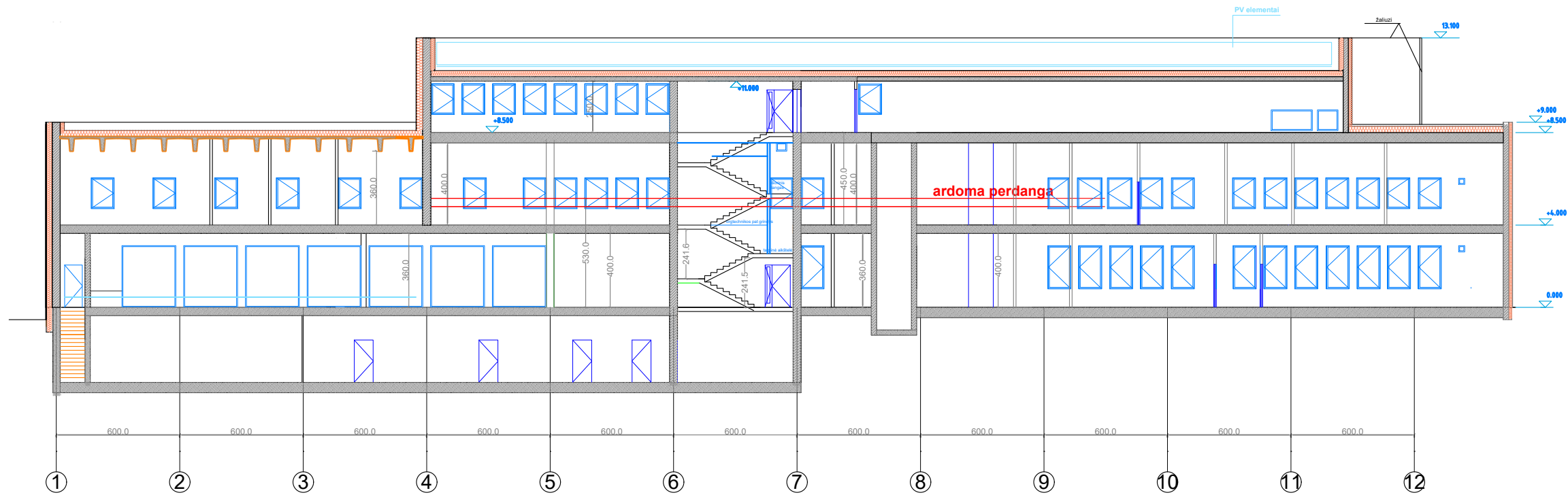
PJŪVIS D-D
