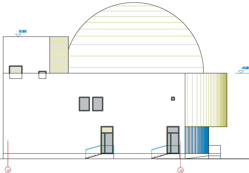
FASADAS H-A
