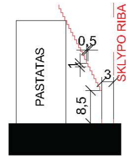
PASTATO AUKŠČIO SKAIČIAVIMO SCHEMA PAGAL STR 2.02.01:2004 "Gyvenamieji pastatai"
