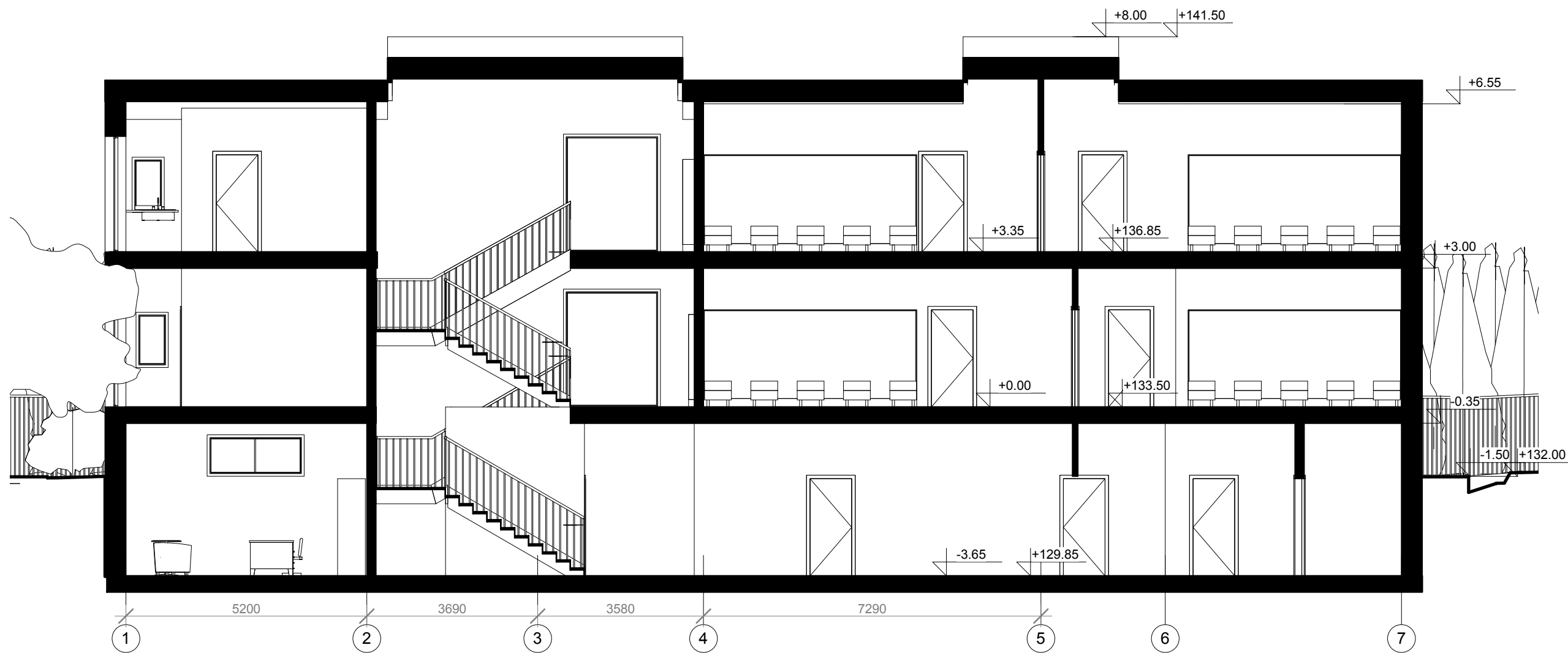
PJŪVIS A-A
