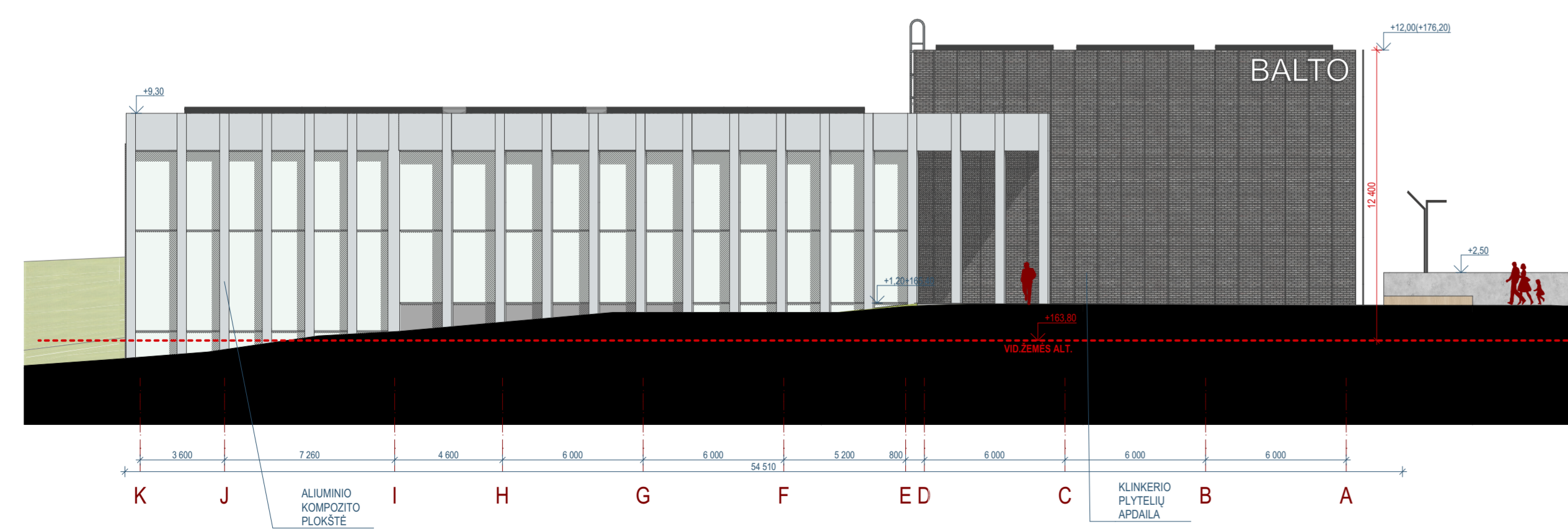
F-03 FASADAS L-A 1:200
