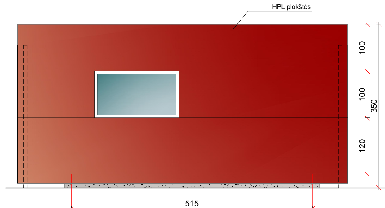
FASADAS AŠYSE 2-1
