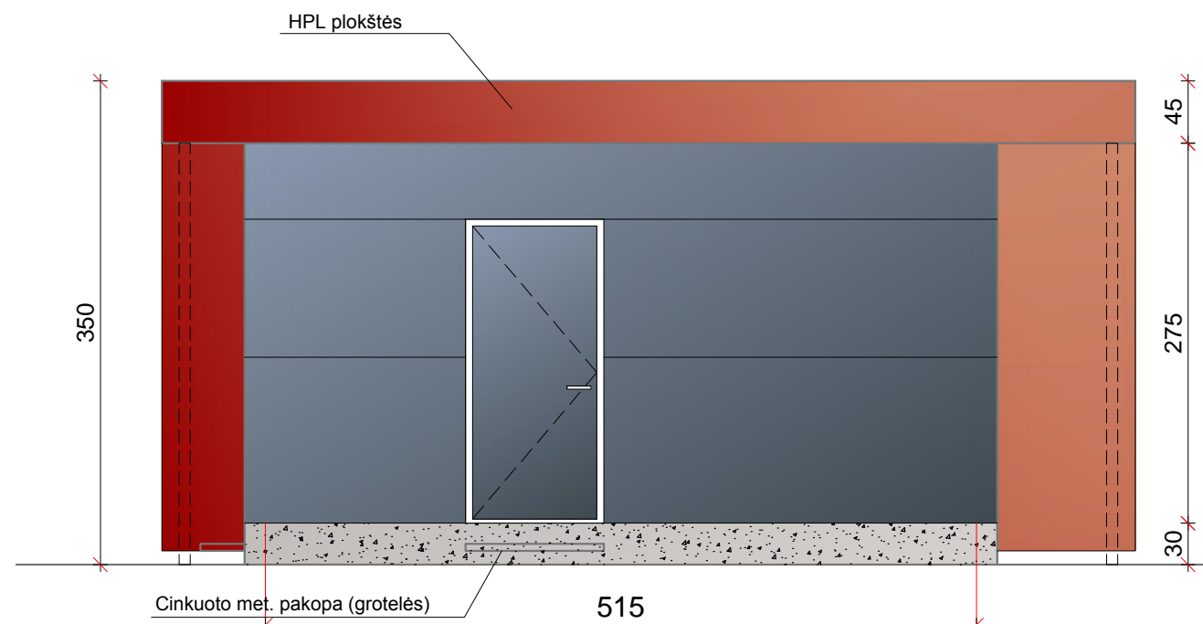
FASADAS AŠYSE 1-2
