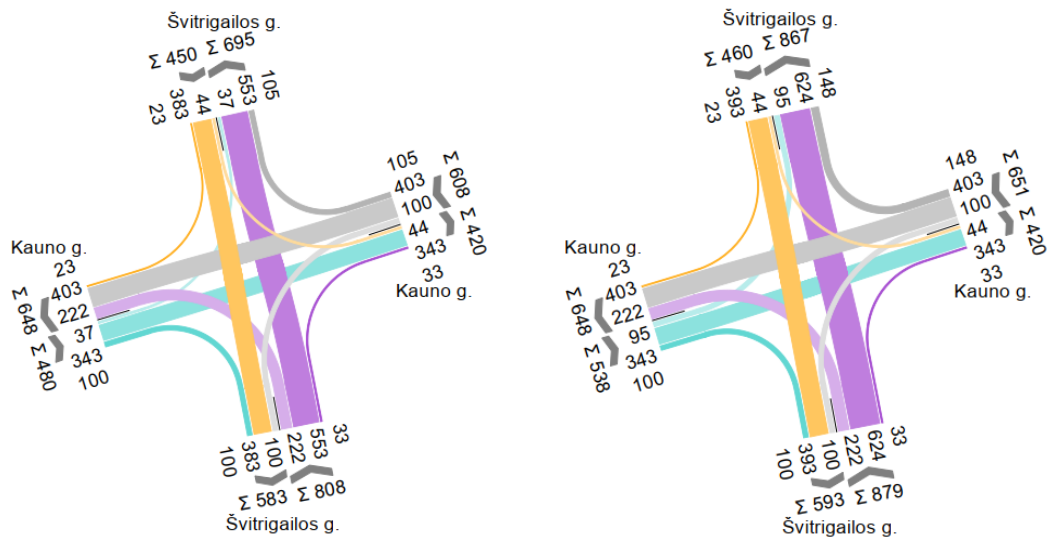
16 pav. Eismo intensyvumai (esami ir perspektyviniai) rytinio piko metu
