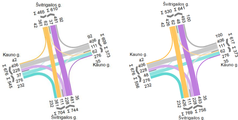
17 pav. Eismo intensyvumai (esami ir perspektyviniai) vakarinio piko metu
