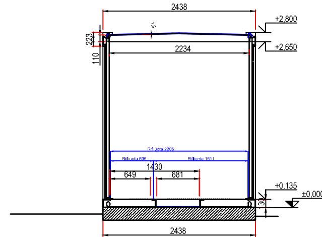
PJŪVIS A-A
