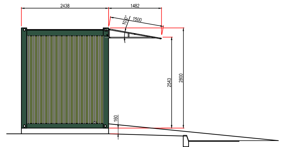
PJŪVIS A-A
