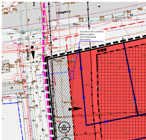
4 pav. ištrauka iš rengiamo detaliojo plano pagrindinio brėžinio
