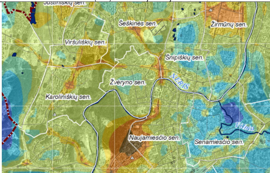
Vidutinė metinė sieros dioksido (SO 2 ) koncentracija (µg/m 3 ) aplinkos ore Vilniuje 2020 m.
