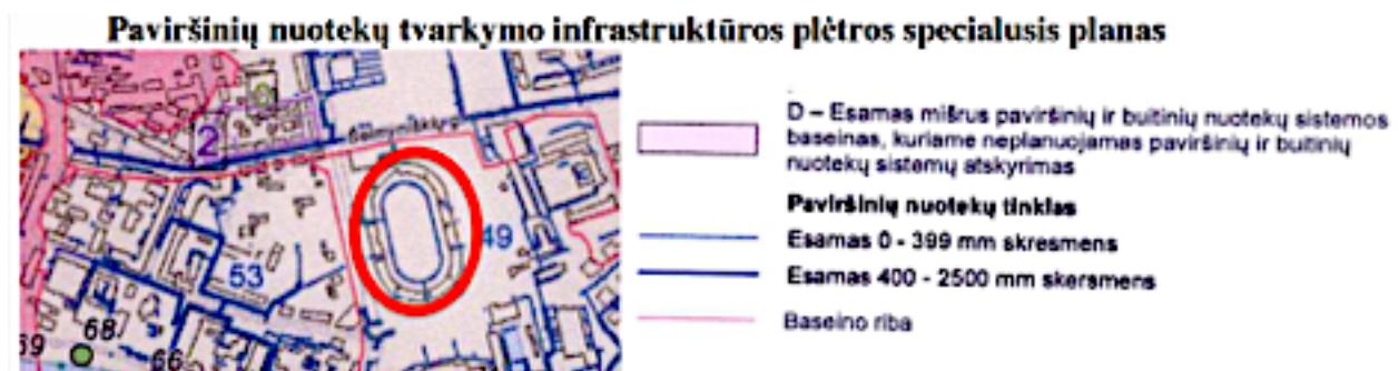
8 pav. Ištrauka iš Paviršinių nuotekų tvarkymo infrastruktūros plėtros specialiojo plano
