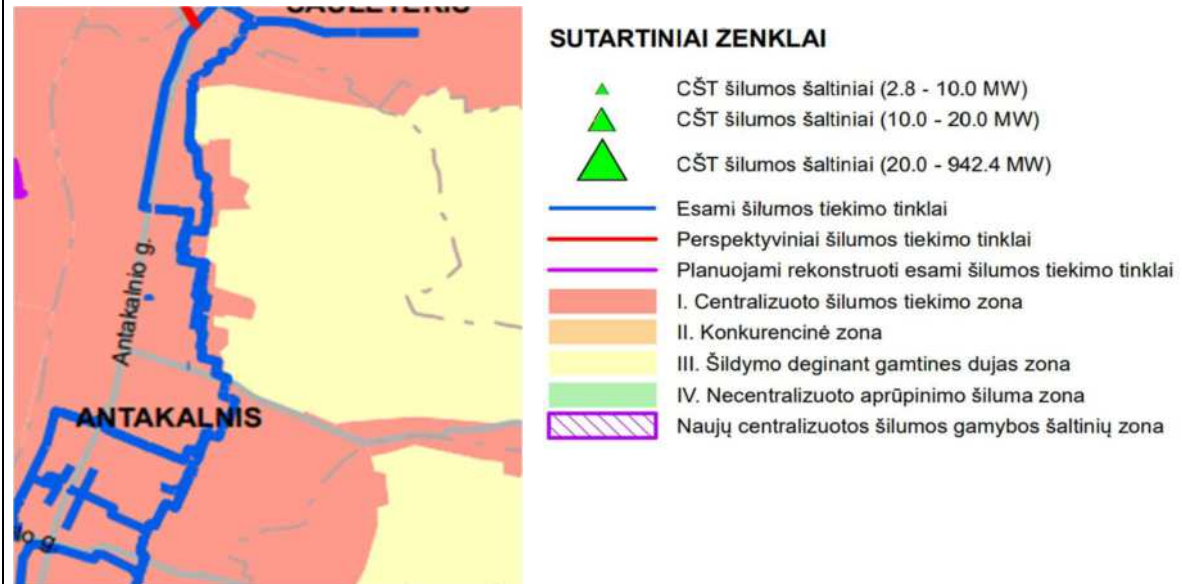
2 pav. Vilniaus miesto savivaldybės teritorijos bendrojo plano ištrauka. Inžinerinė infrastruktūra. Šilumos tiekimas.
