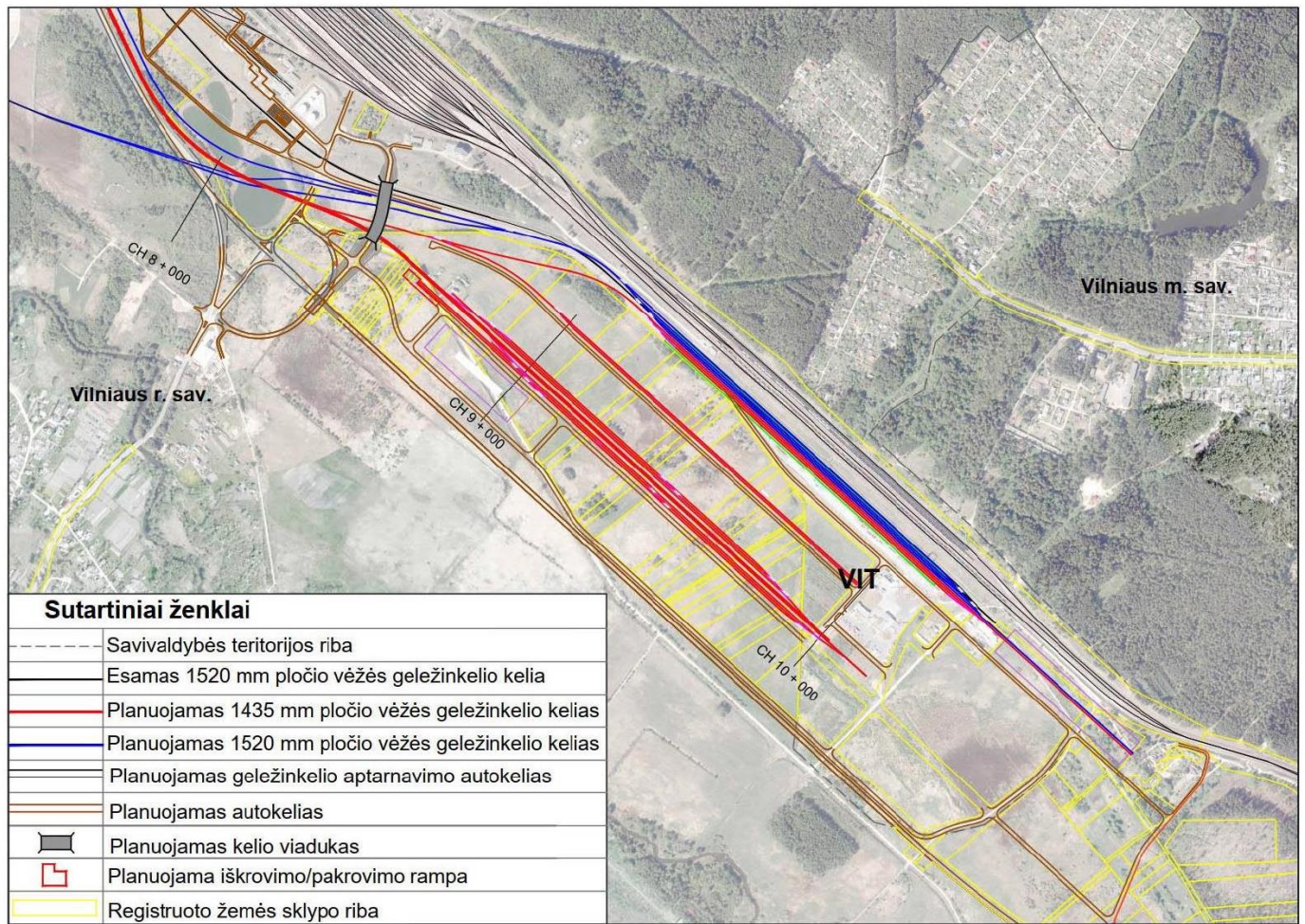
23 pav. VIT krovinų stoties išvystymas (inf. šaltinis - Projekto „Rail Baltica“ geležinkelio linijos Kaunas–Vilnius susisiekimo komunikacijų inžinerinės infrastruktūros vystymo plano aiškinamasis raštas)
