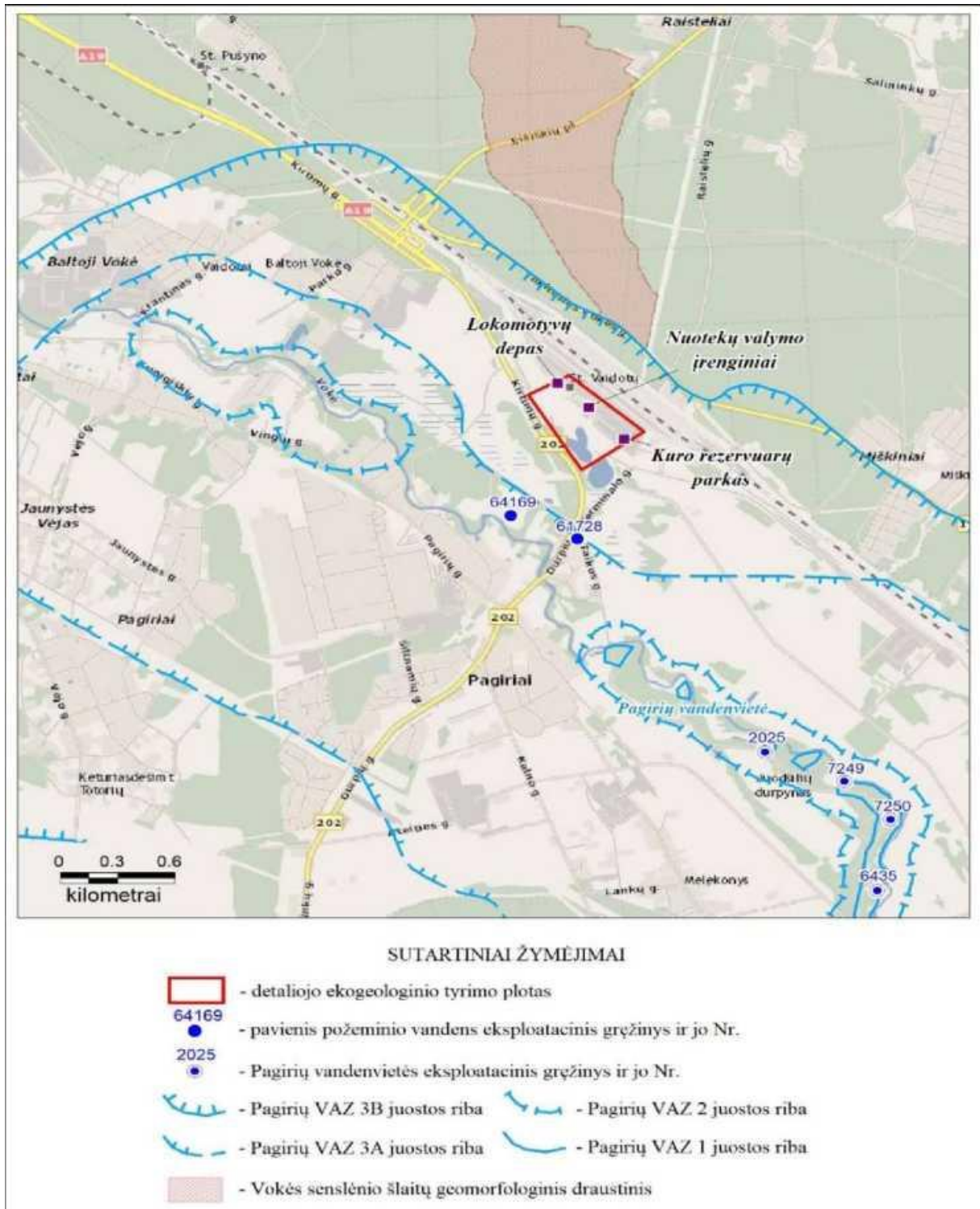
23 pav. Tirtos sklypo padėties schema
