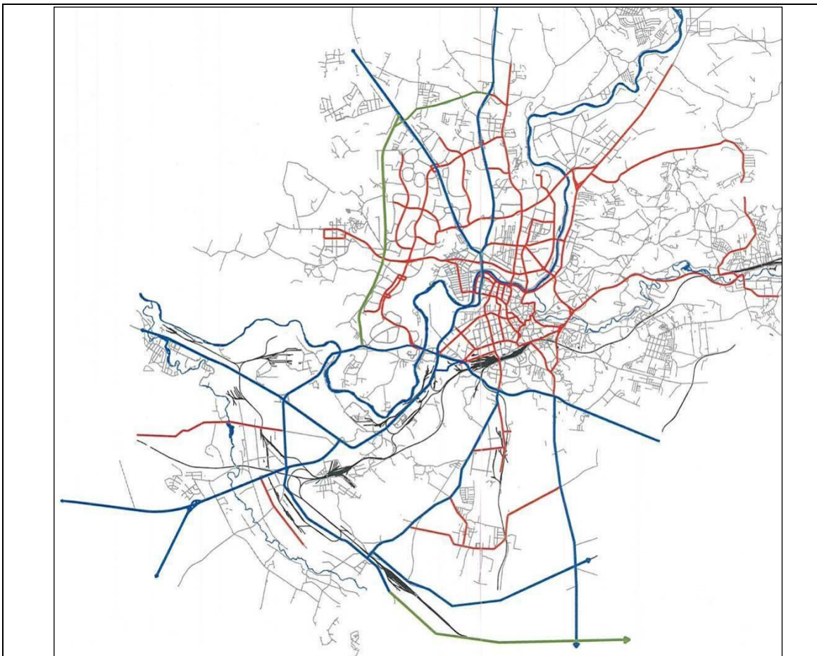
26 pav. Krovininio transporto eismo iš planuojamo Vaidotų logistikos centro Vilniaus miesto teritorijoje principinė eismo schema. (Sutartiniai pažymėjimai: raudonos linijos – magistralinės miesto gatvės nekrovininio transporto eismo iš Vaidotų logistikos centro; mėlynos linijos – pagrindinės esamos krovininio transporto eismo trasos iš Logistikos centro; žalios linijos – pagrindinės perspektyvinės krovininio transporto eismo trasos iš Logistikos centro pagal Vilniaus miesto Bendrojo plano sprendinius (schema panaudota iš 2011 m patvirtinto DP, todėl atkreipiamas dėmesys, kad Vakarinio aplinkkelio sprendiniai jau yra įgyvendinti))
