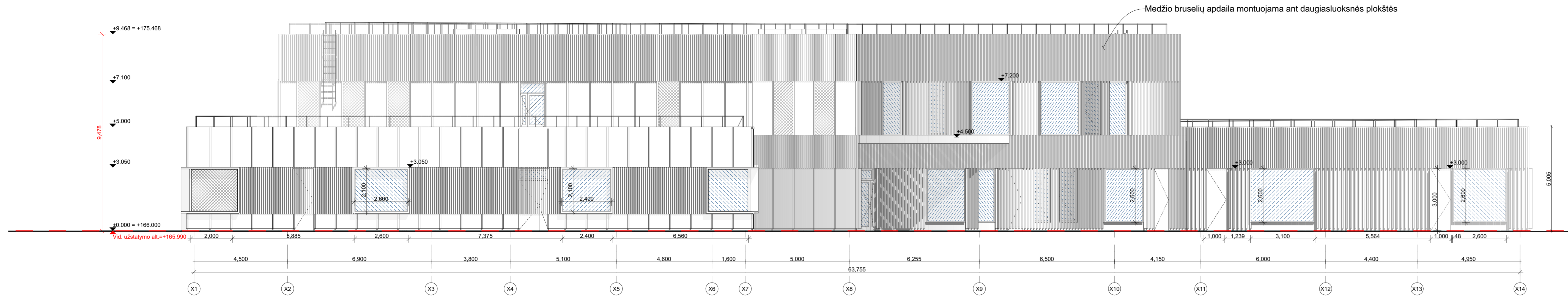
FASADAS X1-X7
