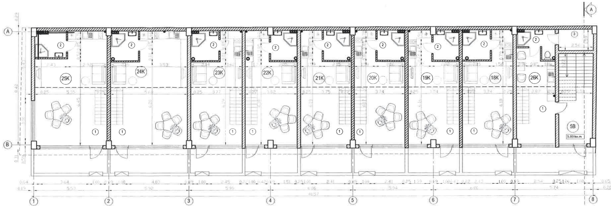
PIRMO AUKŠTO PLANAS M 1:100
