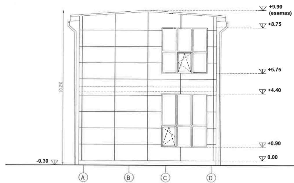
FASADAS TARP AŠIŲ A-D M 1:150
