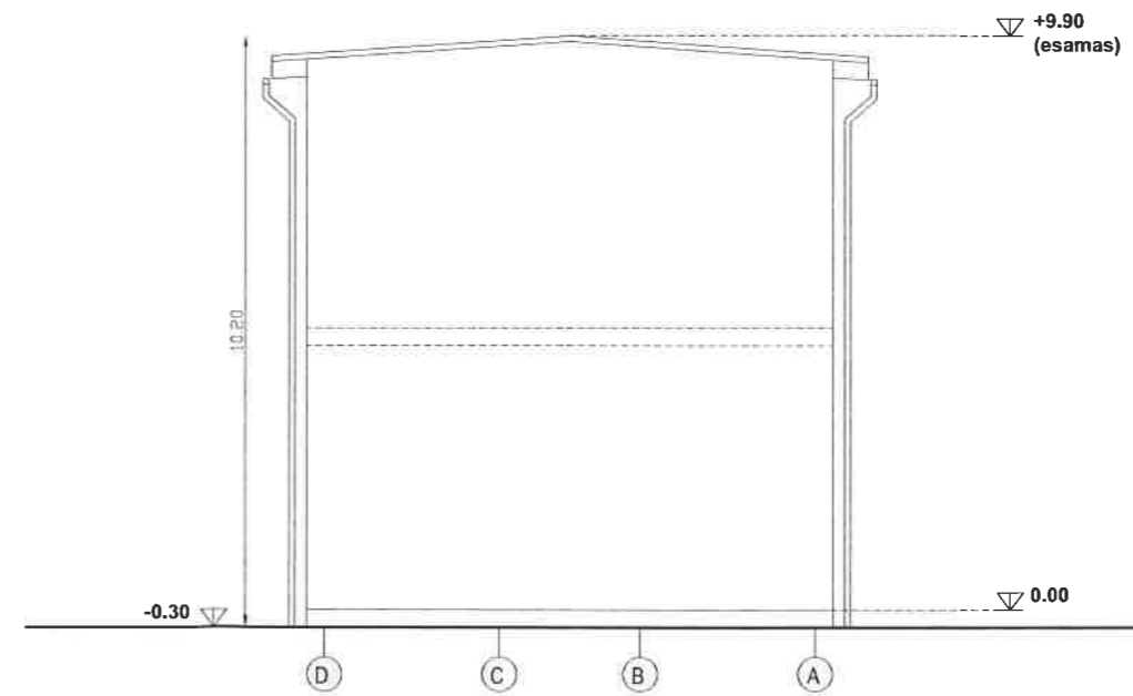
FASADAS TARP AŠIŲ D-A M 1:150
