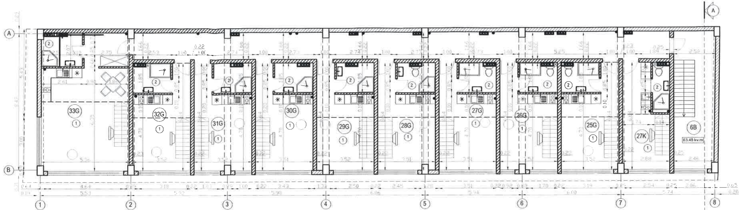
ANTRO AUKŠTO PLANAS M 1:100
