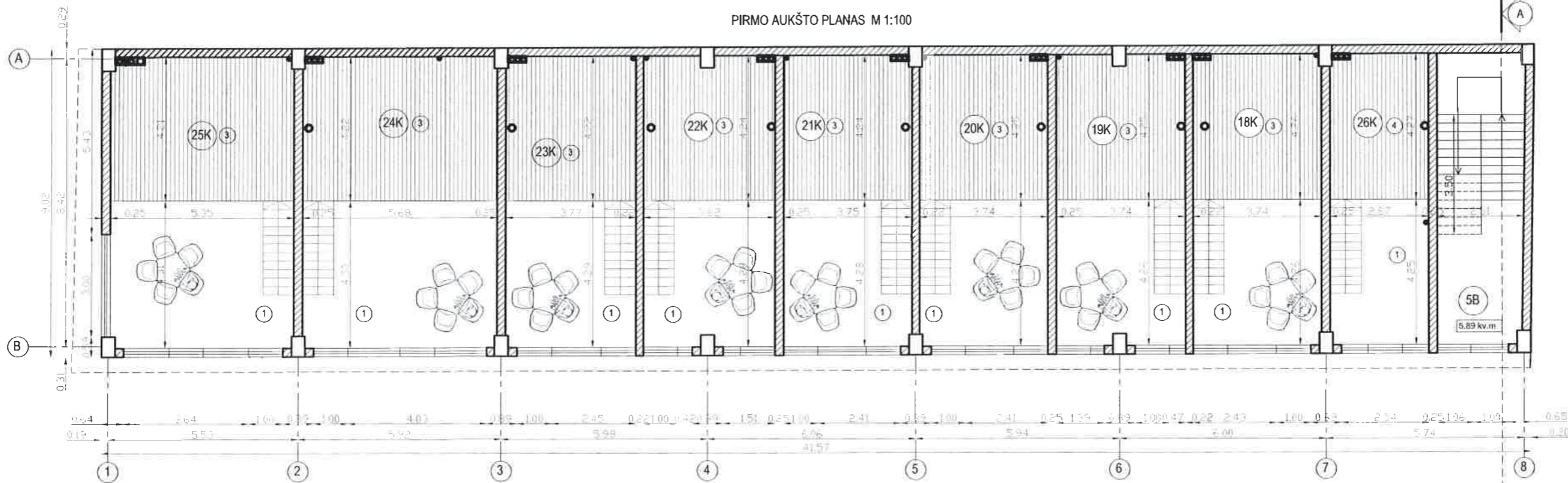
PIRMO AUKŠTO ANTRESOLĖS PLANAS M 1:100
