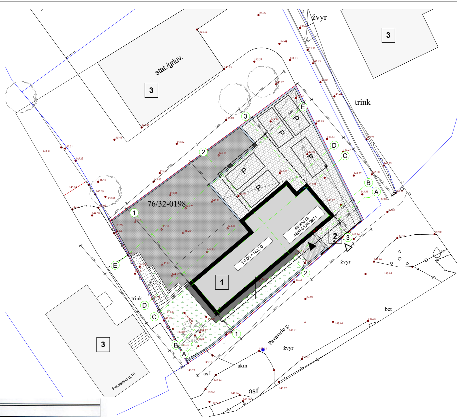
SITUACIJOS SCHEMA
