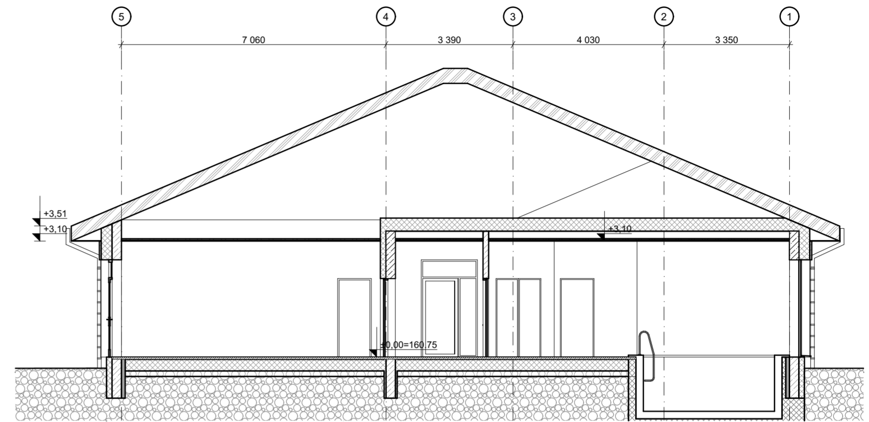
02 PJŪVIS 2-2 1:100
