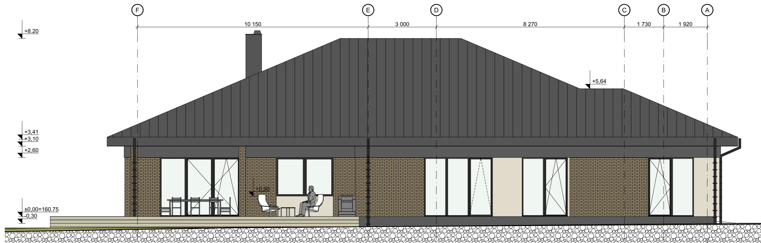
FASADAS TARP AŠIŲ F-A M1:100
