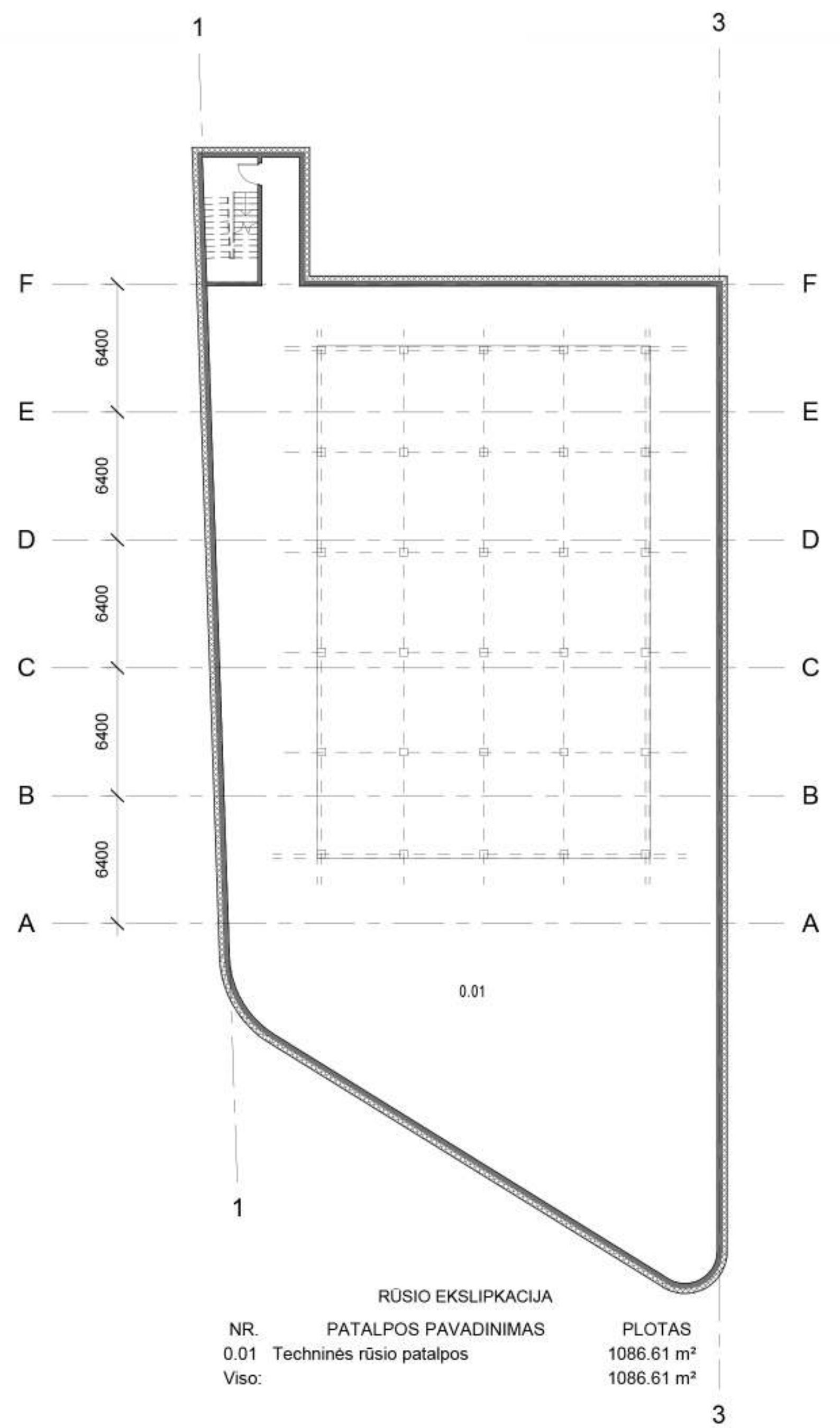
RŪSIO PLANAS M 1:100
