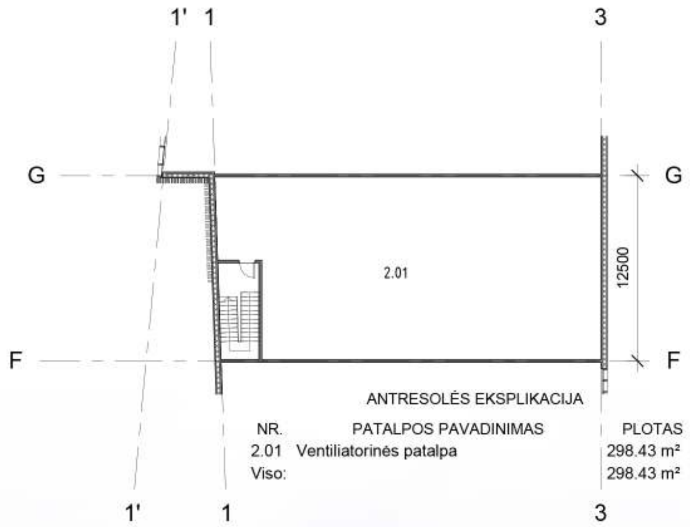
ANTRESOLĖS PLANAS M 1:100
