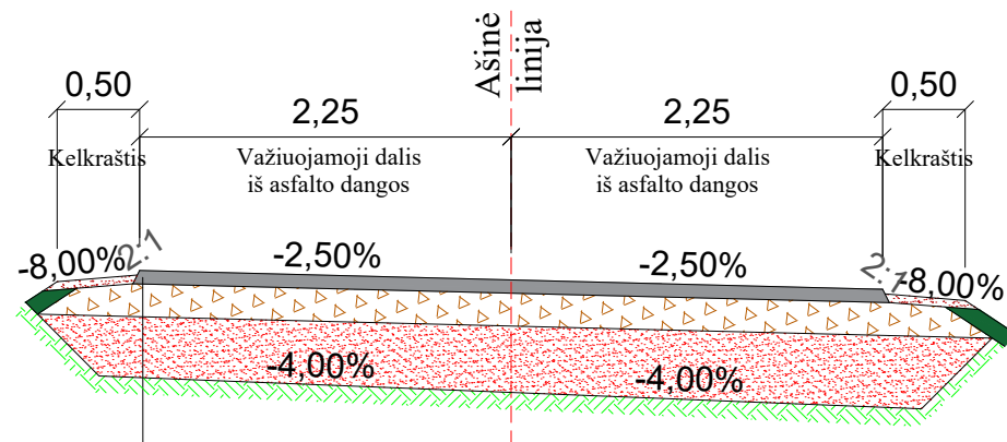
Skersinis pjūvis 1-1
