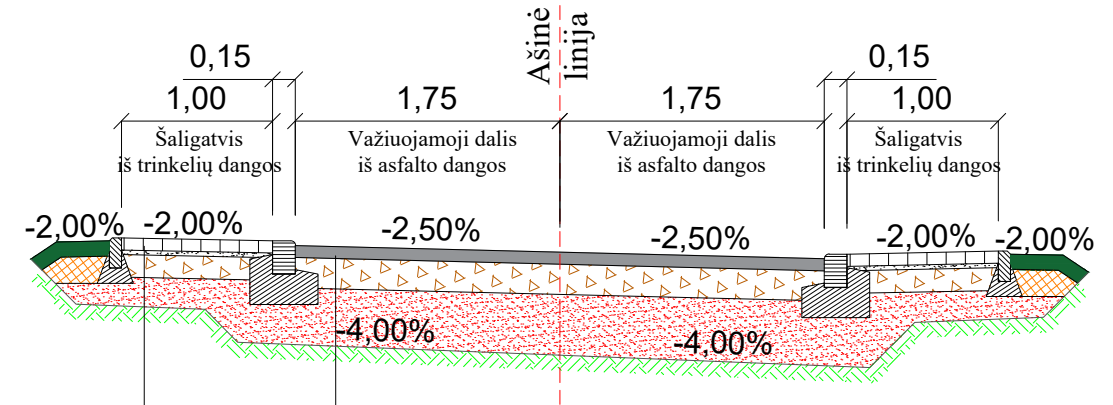
Skersinis pjūvis 2-2
