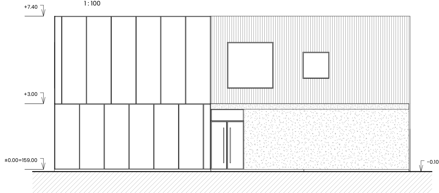
VAKARINIS FASADAS 1:100
