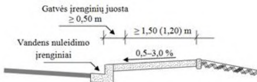
Brėžinys nr. 1 Tipinis pėsčiųjų tako (šaligatvio) skersinis profilis
