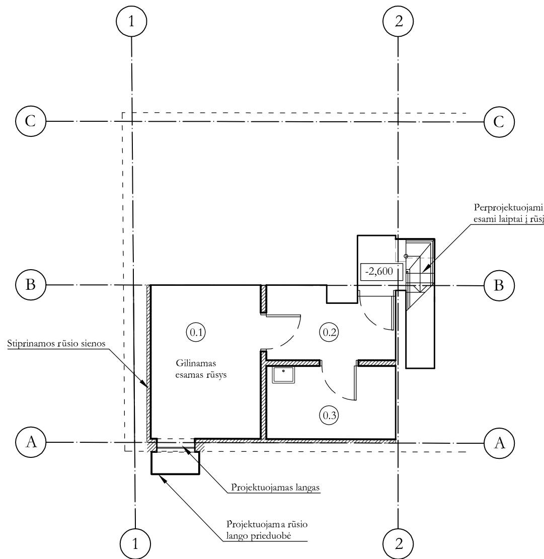
Rūšio planas M 1:100
