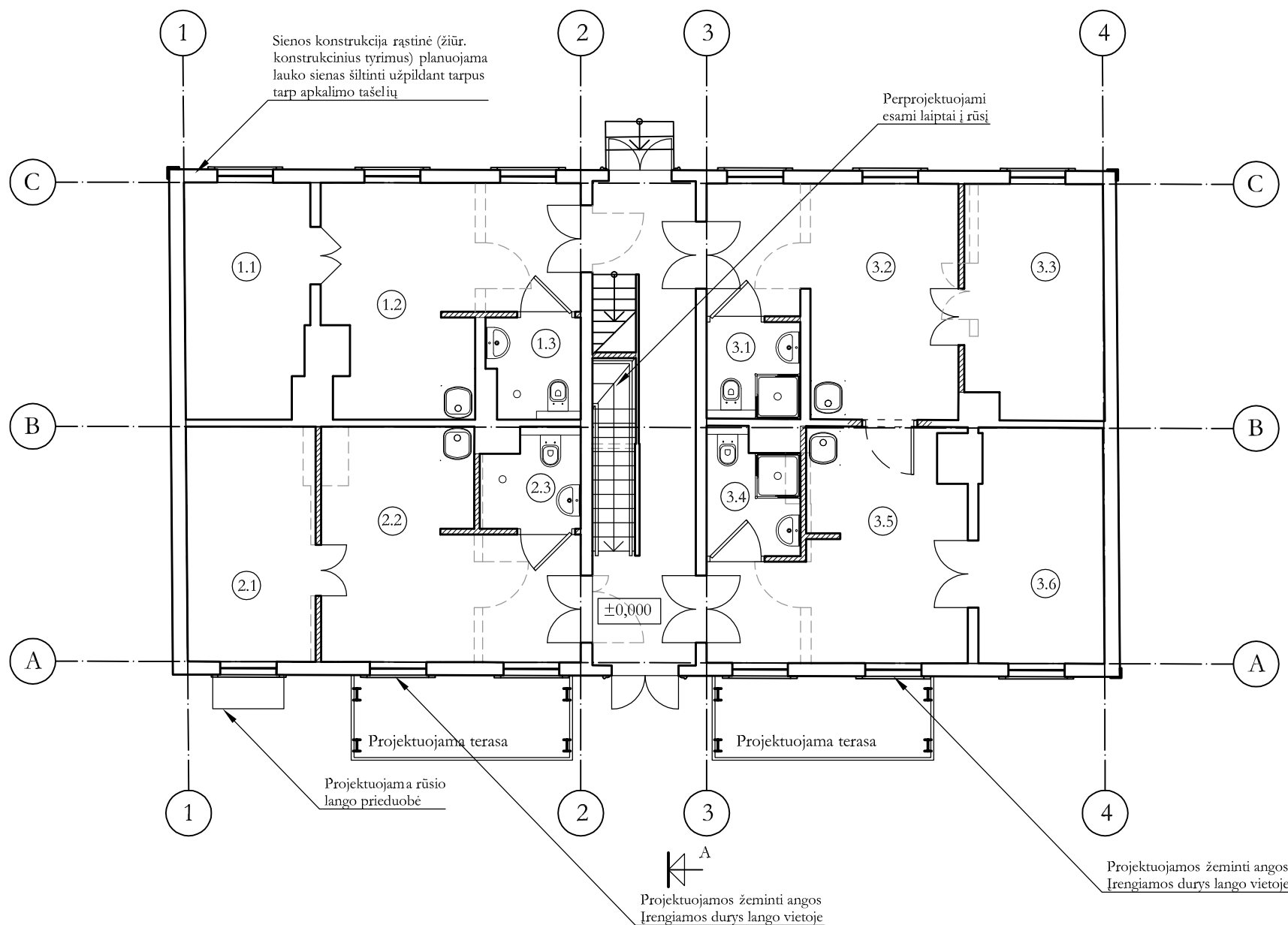
Pirmo aukšto planas M 1:100
