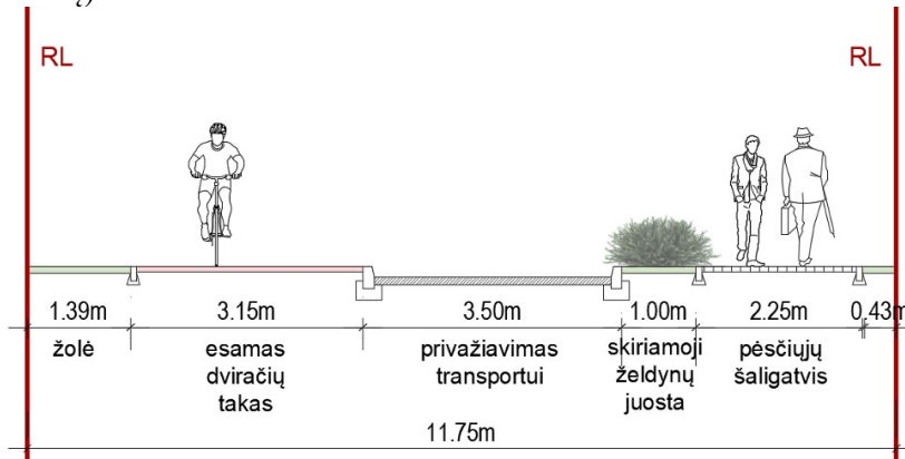
2 pav. Rekomendacinis Neries g. pjūvis su siūlomu privažiuoimu specialiajam ir aptarnaujančiam transportui
