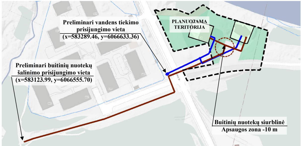
4 pav. Rekomendacinio pobūdžio inžinerinių tinklų schema
