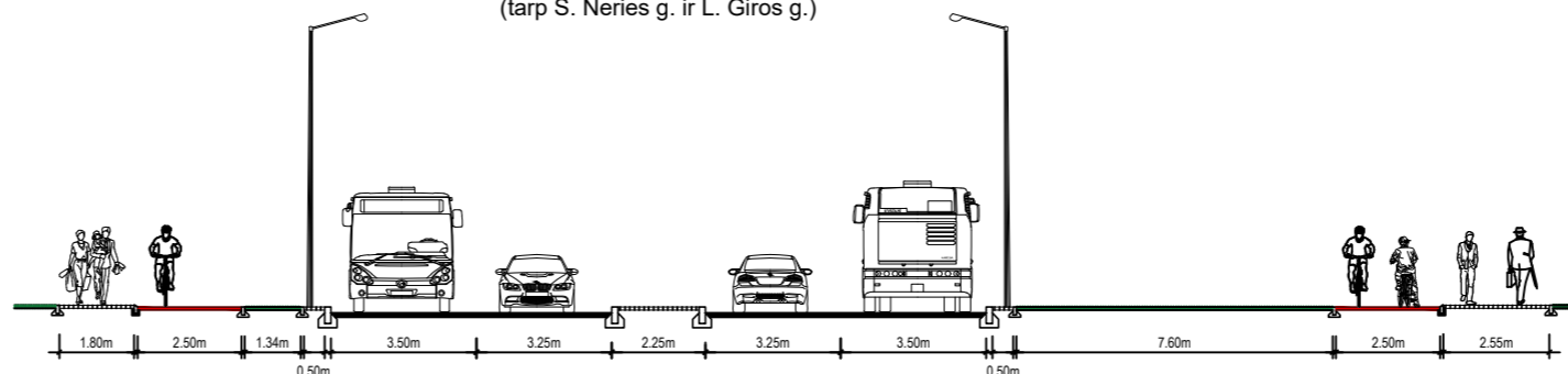
Pjūvis 6 - 6 L. Zamenhofo g. (tarp S. Neries g. ir L. Giros g.)
