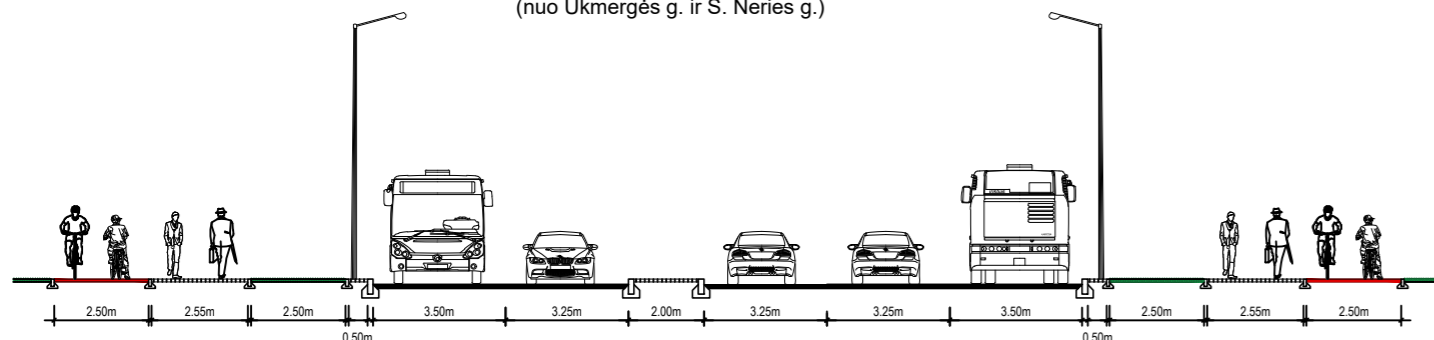
Pjūvis 5 - 5 L. Zamenhofo g. (nuo Ukmergės g. ir S. Neries g.)
