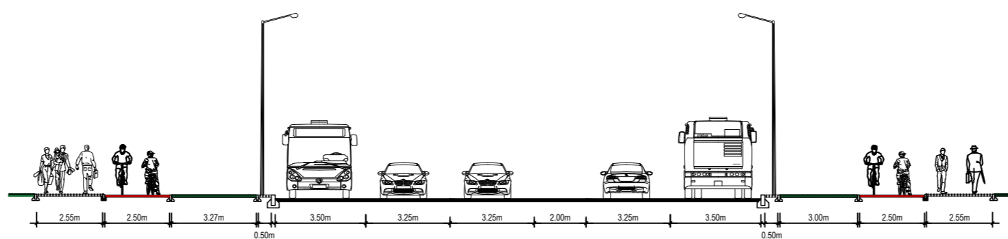
Pjūvis 2 - 2 Pavilionių g. (tarp Perkūnkiemo ir Justiniškių g.)
