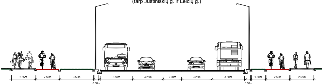
Pjūvis 3 - 3 Pavilionių g. (tarp Justiniškių g. ir Leičių g.)
