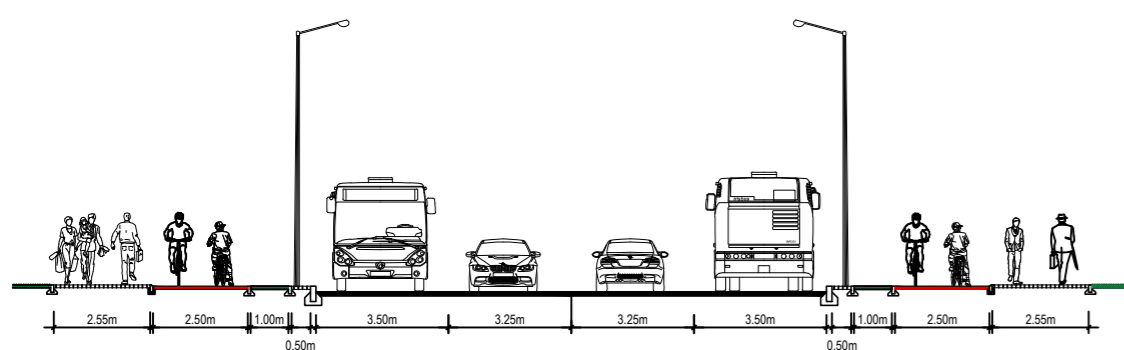
Pjūvis 1 - 1 Pavilionių g. (tarp Vakarinio aplinkkelio ir Perkūnkiemo g.)
