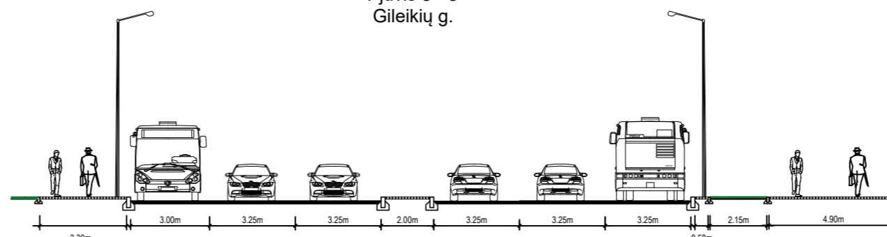
Pjūvis 8 - 8 Gileikių g.
