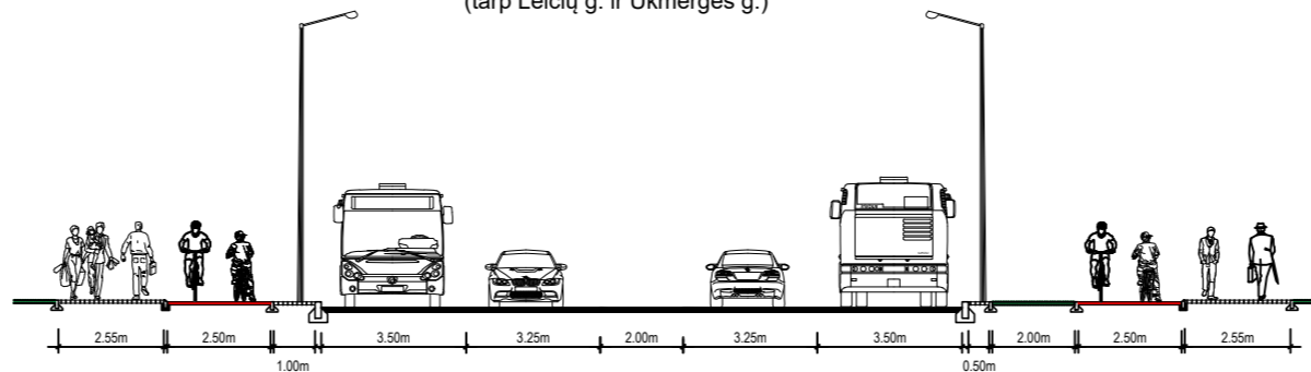
Pjūvis 4 - 4 Pavilionių g. (tarp Leičių g. ir Ukmergės g.)
