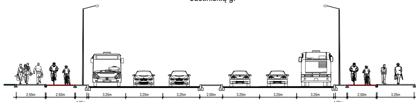
Pjūvis 7 - 7 Justiniškių g.
