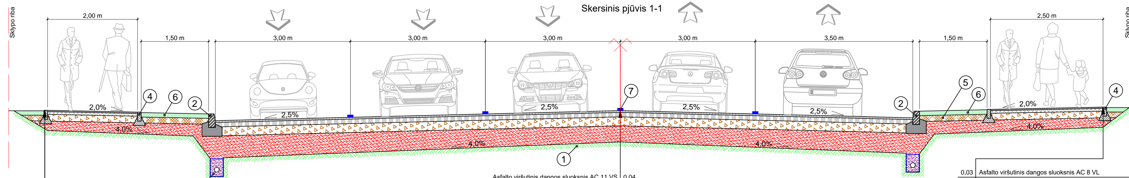
Skersinis pjūvis 1-1
