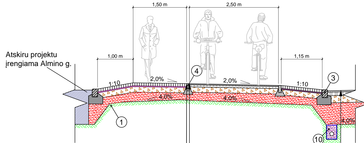
Skersinis pjūvis 4-4
