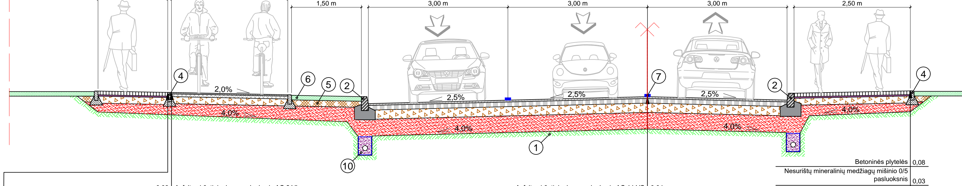
Skersinis pjūvis 3-3
