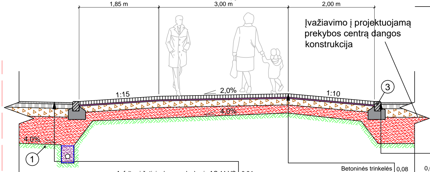
Skersinis pjūvis 2-2
