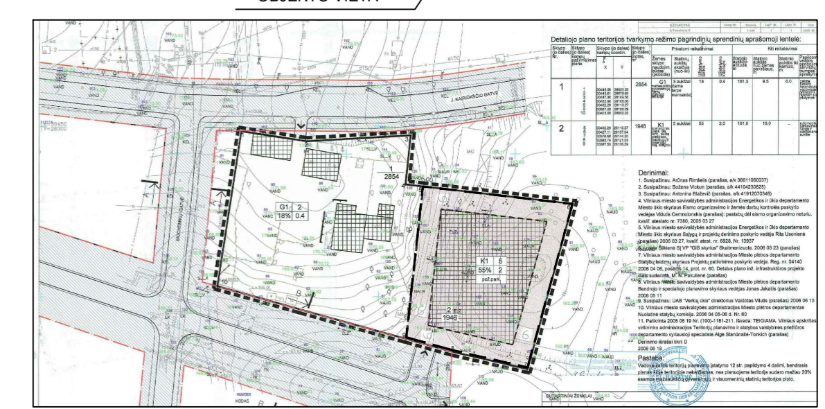
IŠTRAUKA IŠ ŽEMĖS SKLYPO J. KAIRIŪKŠČIO G. 3 (KAD.NR. 0101/0004:132)-0,48 HA DETALIOJO PLANO
