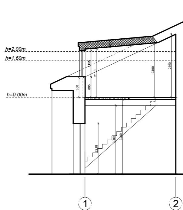
PJŪVIS 2-2, M1:100
