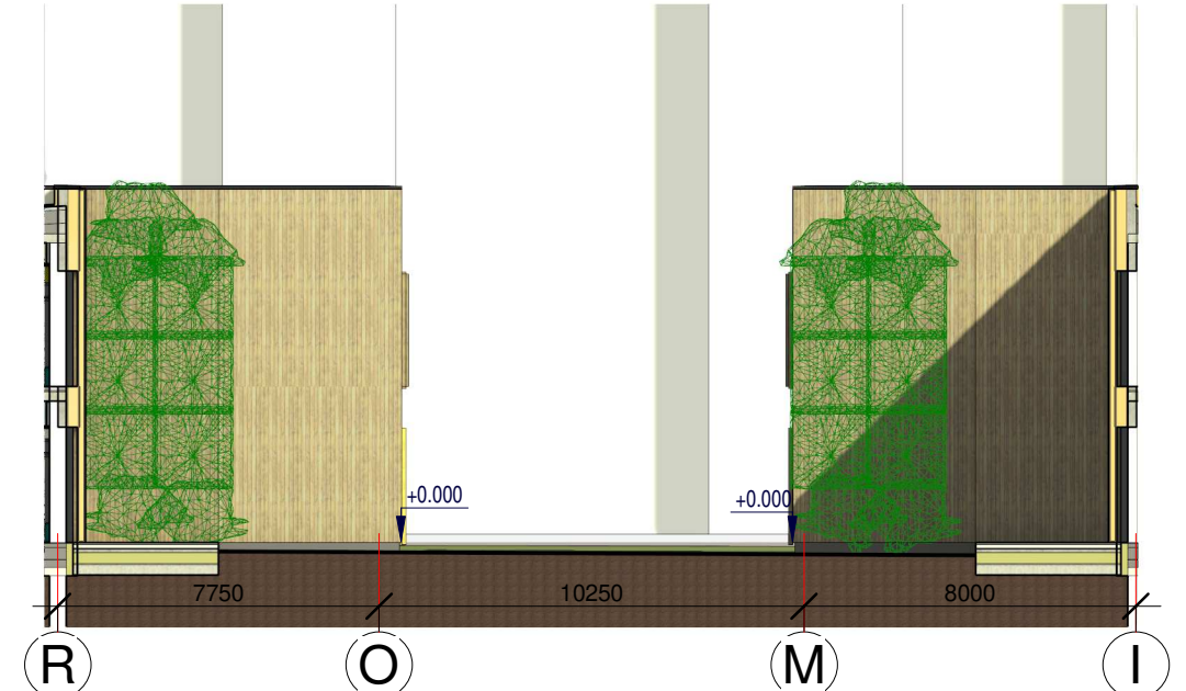
4 Išklotinė R-I 1 : 200
