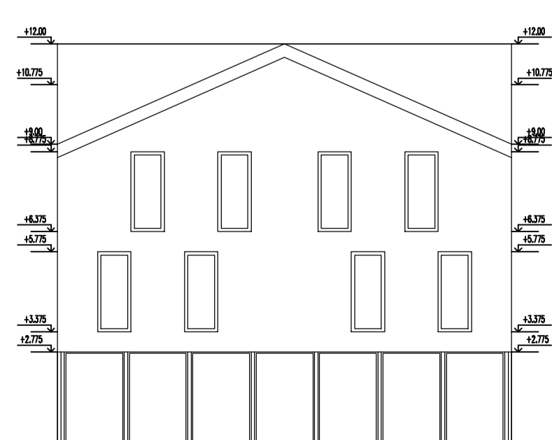
40 4-5-6 korpusų Pietų fasadas
