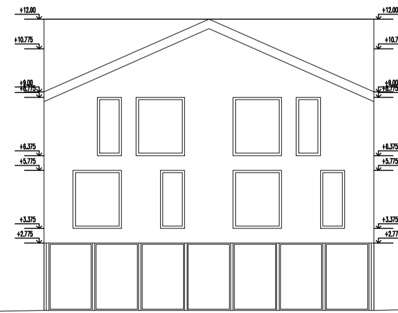
40 5,6,8 korpusų Šiaurės fasadas
