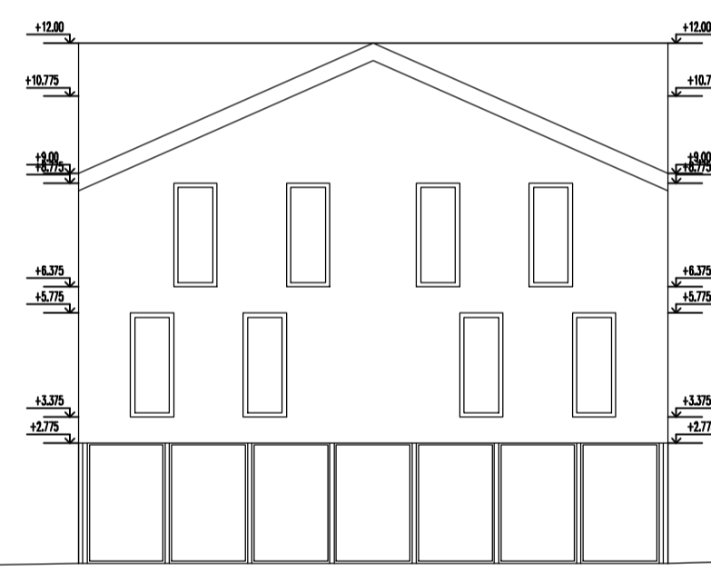
40 1-2-3 korpusų Šiaurės fasadas
