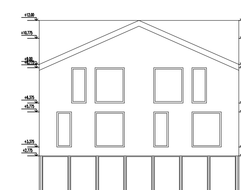
40 1-2-3 korpusų Pietų fasadas
