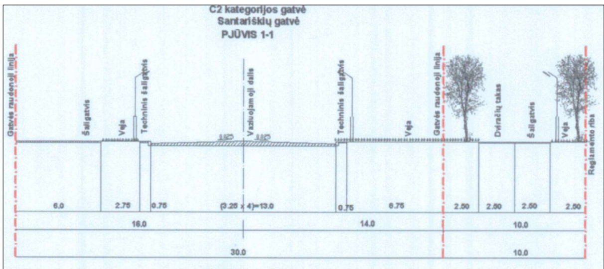
16 pav. C2 gatvės kategorijos pjūvis.
