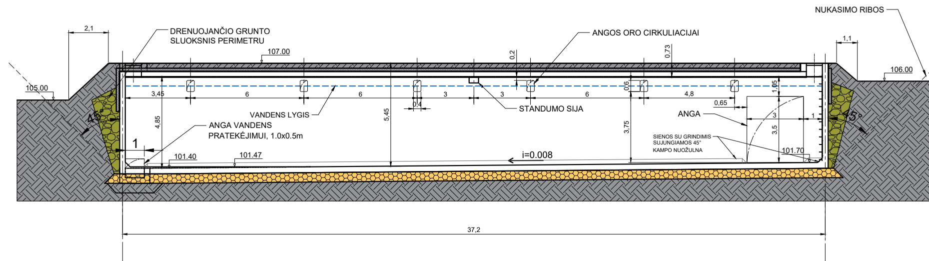
REZERVUARO IŠILGINIS PJŪVIS M 1:200
