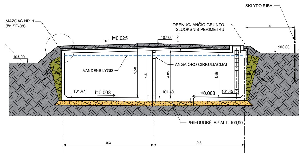
REZERVUARO SKERSINIS PJŪVIS M 1:200
