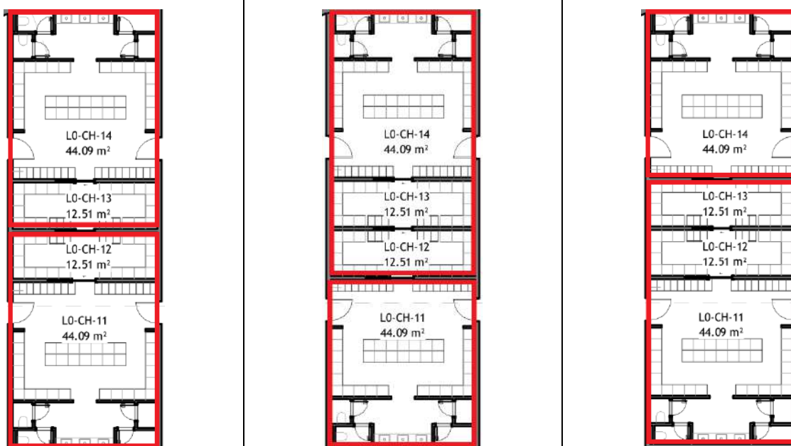
Pav. 17. Grupinių persirengimo kambarių ploto, skirto vyrams-moterims, transformacijos galimybės Group changing rooms. Transformation options
