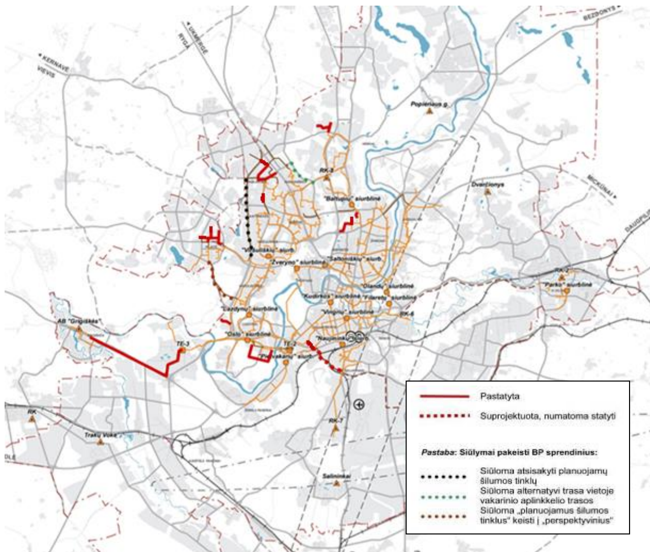
4.9.4.1 pav. Šilumos tiekimo plėtra 2007-2014 m.
