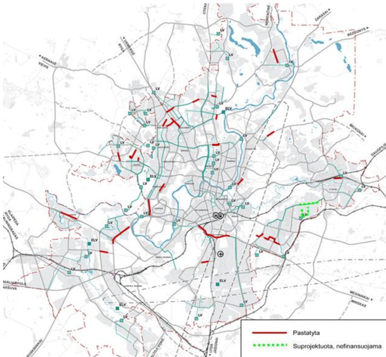
4.9.2.1 pav. Lietaus nuotekynės plėtra 2007-2014 m.
