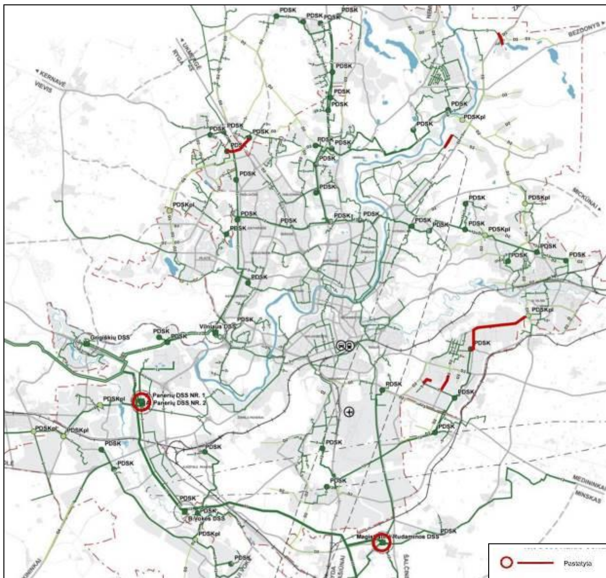
4.9.4.1 pav. Dujotiekio plėtra 2007-2014 m.
