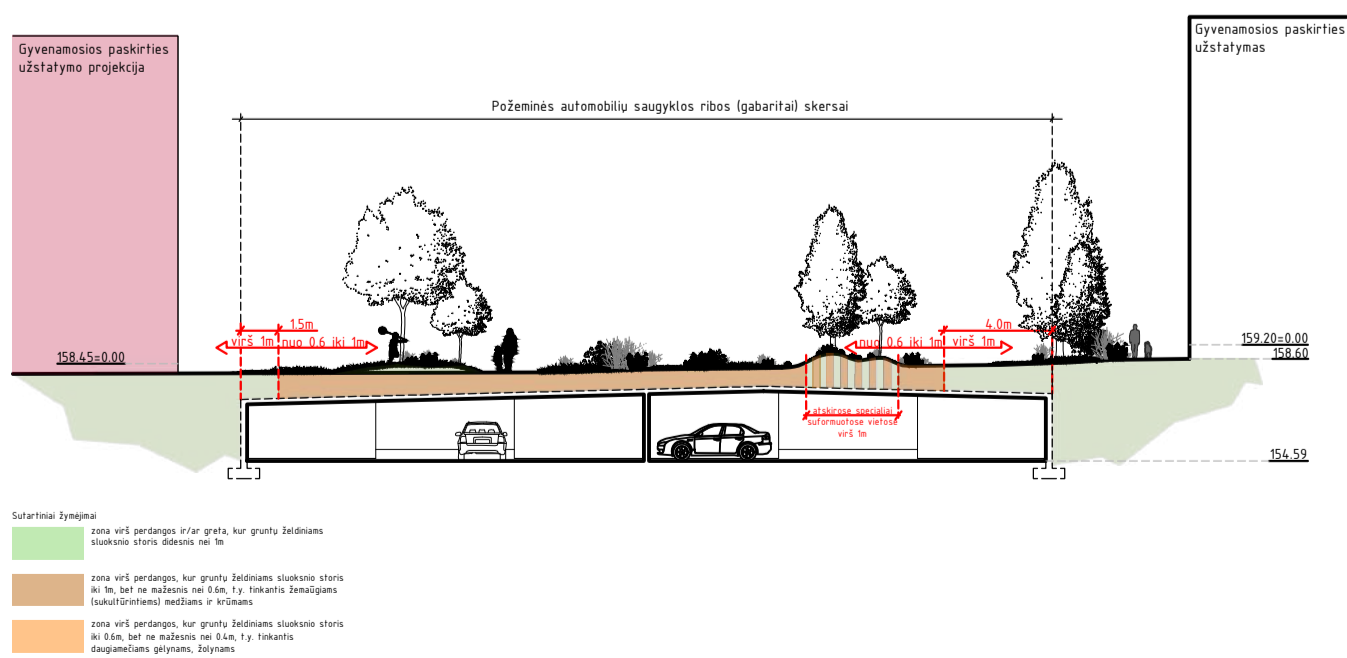
Principinis pjūvis A-A Grunto sluoksnio virš požeminės automobilių saugyklos įvertinimui
