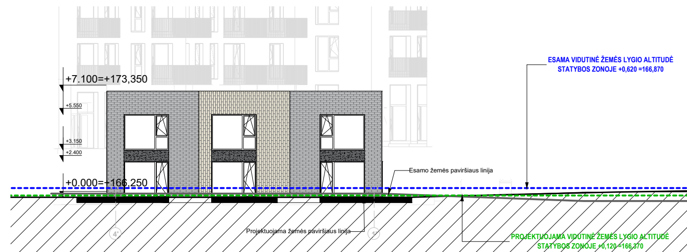
Pjūvis 10-10
