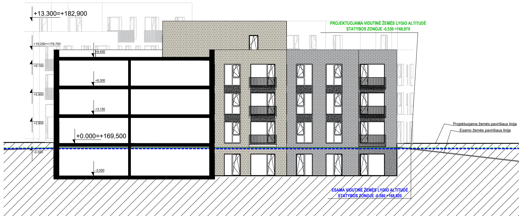
Pjūvis 8-8
