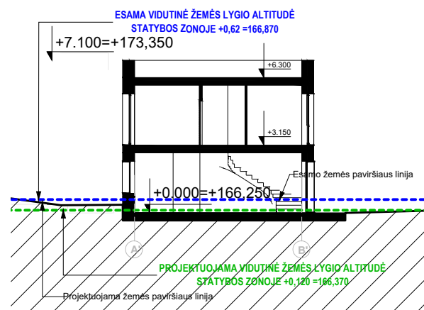
Pjūvis 11-11
