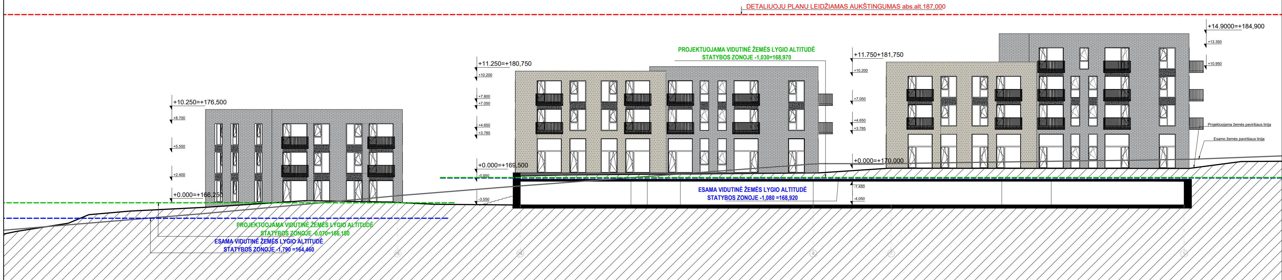
Pjūvis 6-6
