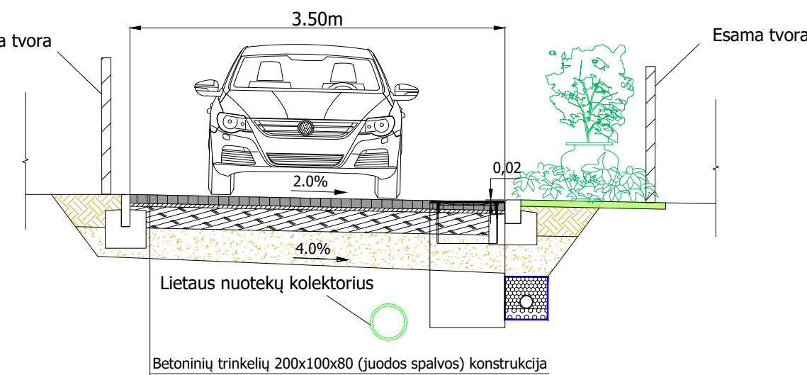
Konstrukcija Kazbėjų g. nuo Pk 0+00 iki Pk 6+52 ties susiaurėjimais Mišraus eismo zona
