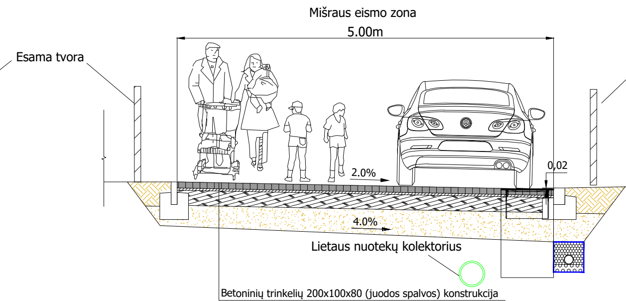
Konstrukcija Kazbėjų g. nuo Pk 0+00 iki Pk 6+52 be gatvių eksploataavimo juostų
