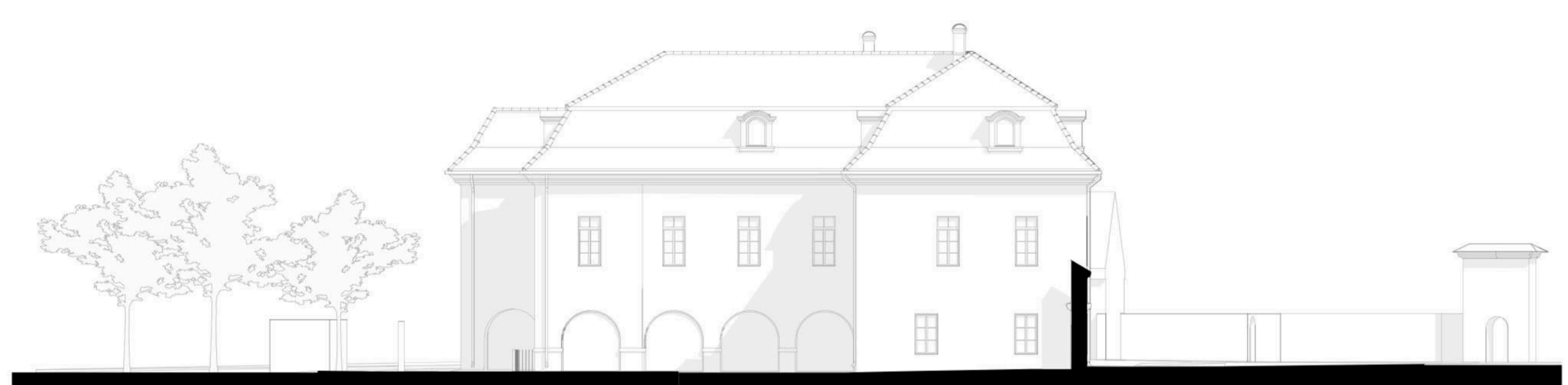
VAKARINIS FASADAS M 1:200
