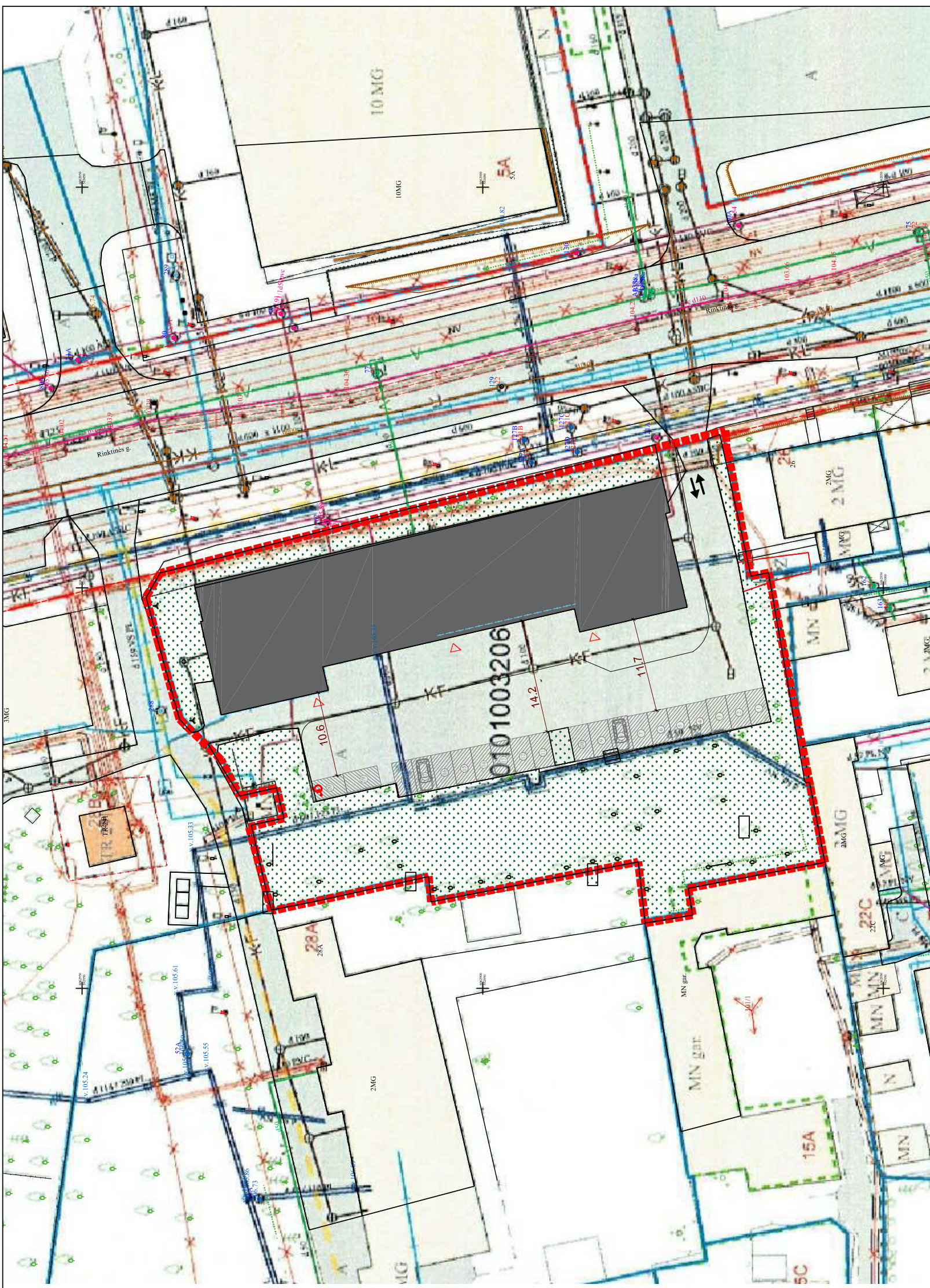
SKLYPO PLANAS M1:500
