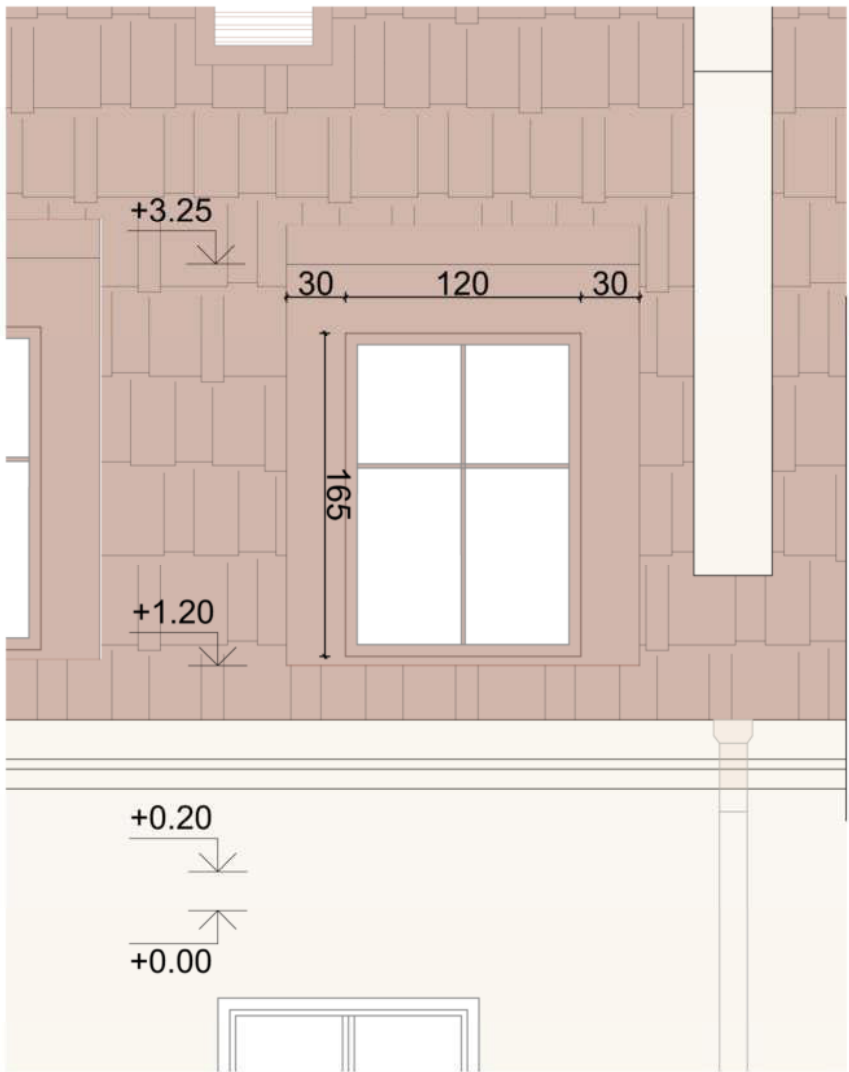
TŪRINIS STOGLANGIS M1:20
