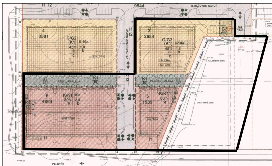
15 pav. Ištrauka iš Pilaitės teritorijos šiaurinės dalies detaliojo plano korektūros brėžinio.
