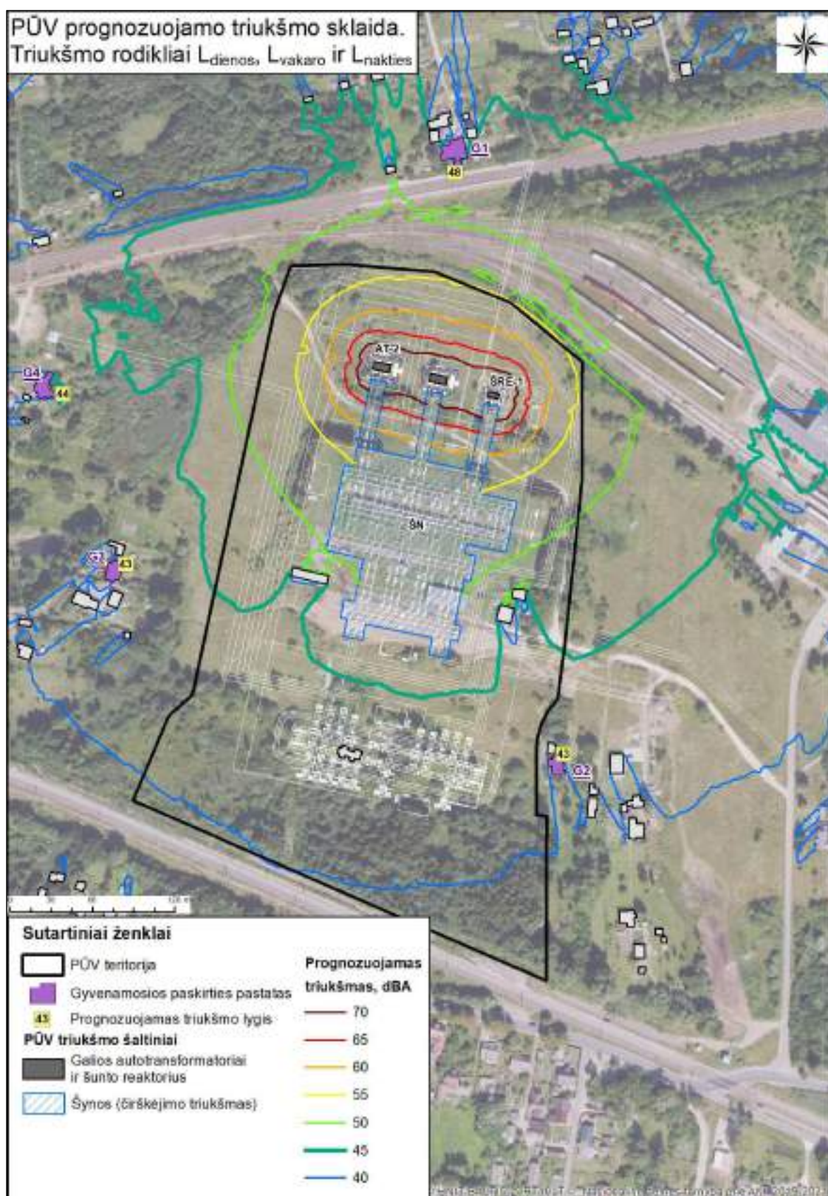
7.2.2.4 pav. Prognozuojamo planuojamos Vilnios TP įrenginių triukšmo sklaida (nakties periodu).
