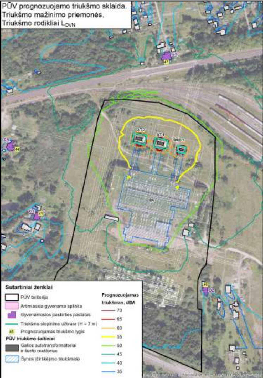
7.2.2.7 pav. Prognozuojamo planuojamos Vilnios TP triukšmo sklaida įvertinus PŪV triukšmo mažinimo priemones (paros periodu)
