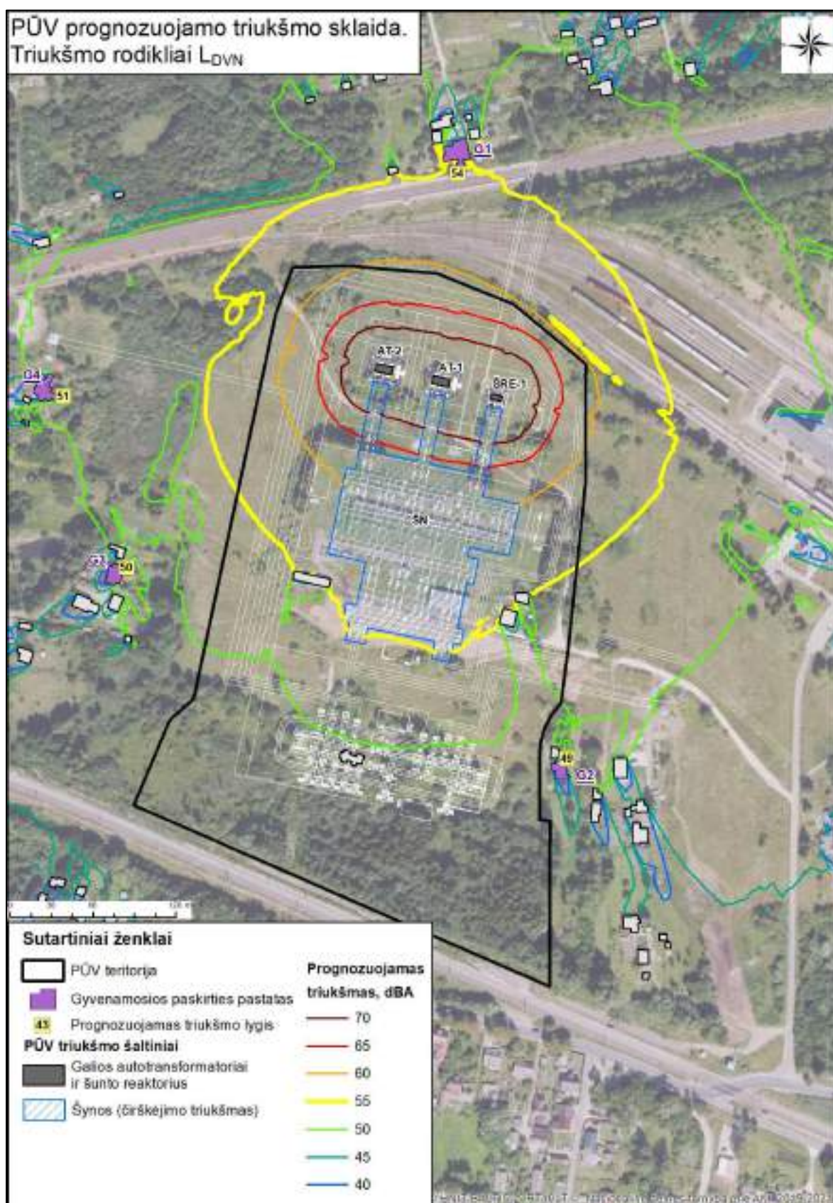
7.2.2.5 pav. Prognozuojamo planuojamos Vilnios TP įrenginių triukšmo sklaida (paros periodu).
