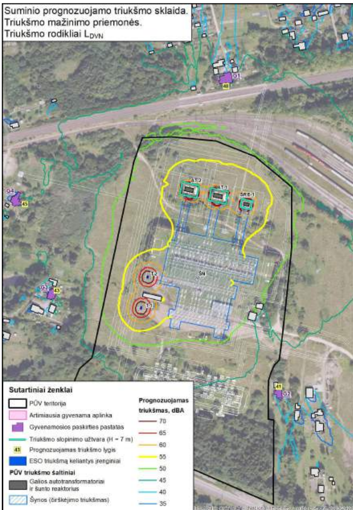
7.2.2.9 pav. Prognuozuojamo planuojamos Vilnios TP ir esamų galios transformatorių suminio triukšmo sklaida įvertinus PŪV triukšmo mažinimo priemones (paros periodu).
