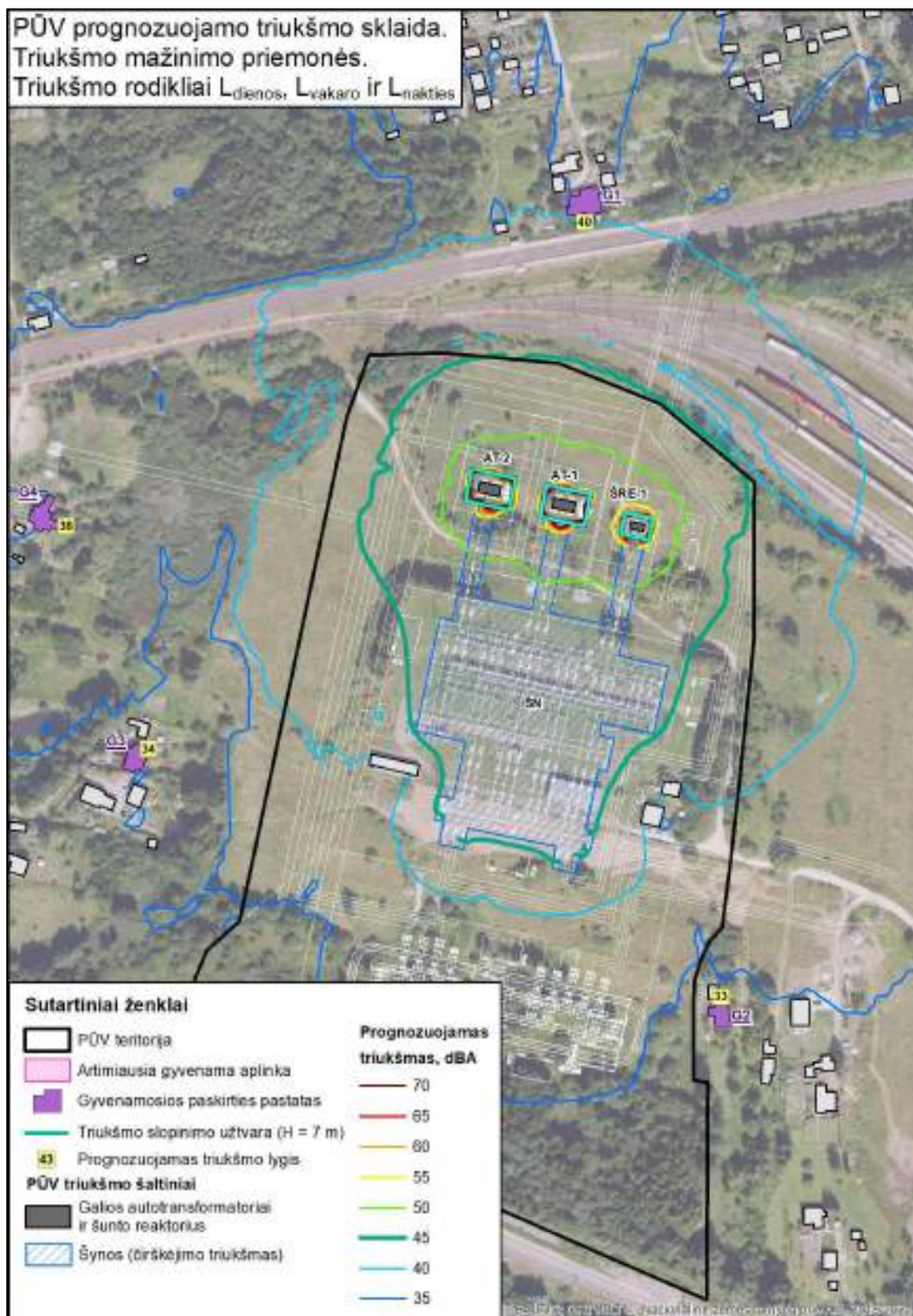
7.2.2.6 pav. Prognozuojamo planuojamos Vilnios TP triukšmo sklaida įvertinus PŪV triukšmo mažinimo priemones (nakties periodu)
