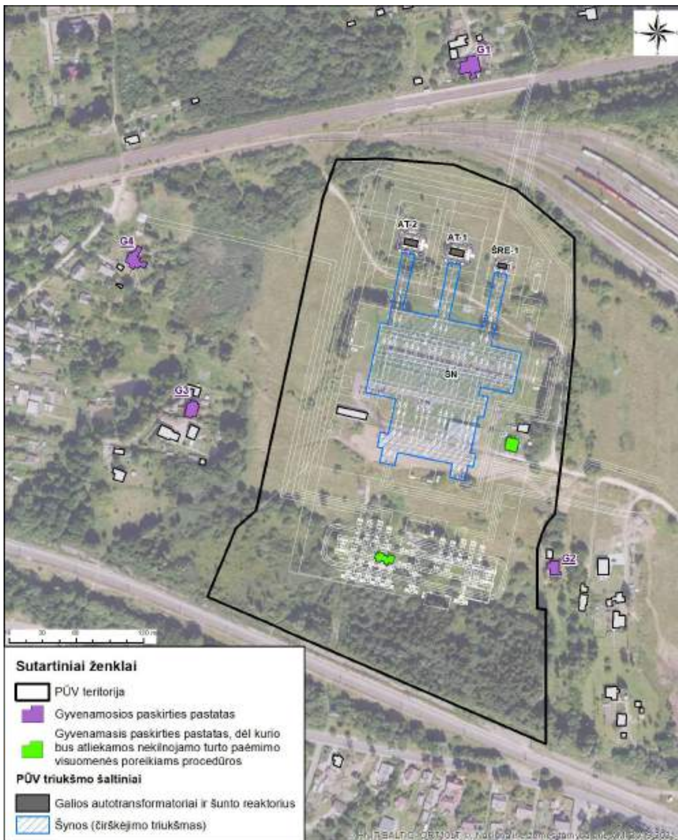
7.2.2.3 pav. Planuojamos Vilnios TP triukšmo šaltinių išdėstymo schema.
