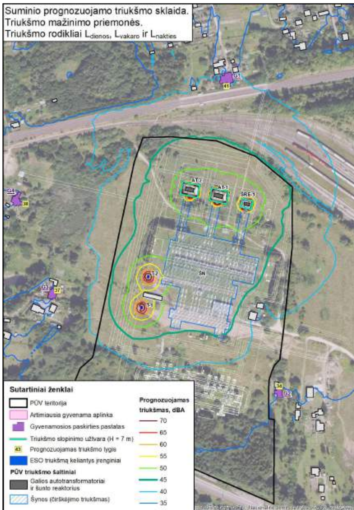
7.2.2.8 pav. Prognozuojamo planuojamos Vilnios TP ir esamų galios transformatorių suminio triukšmo sklaida įvertinus PŪV triukšmo mažinimo priemones (nakties periodu).
