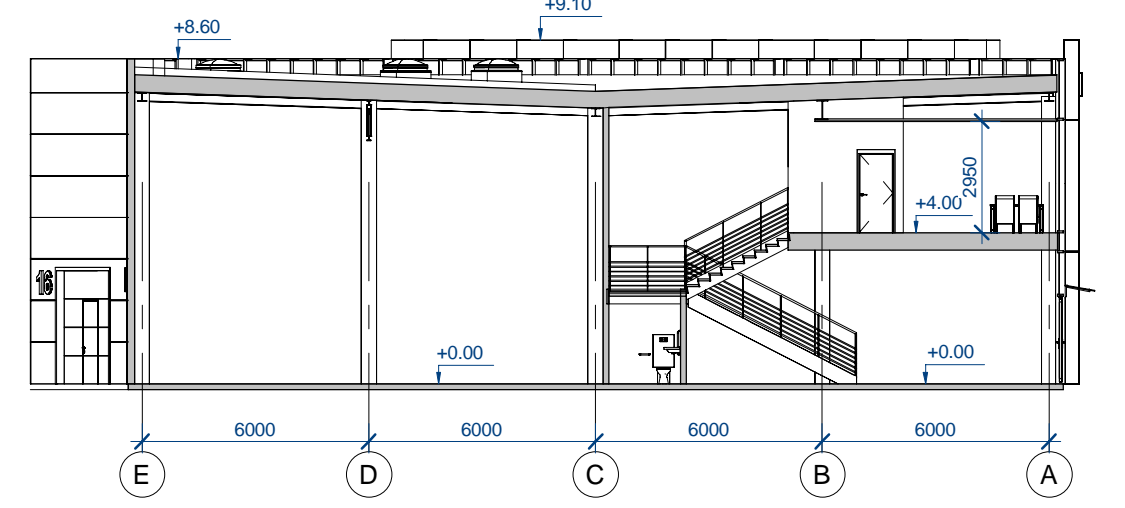
Pijvis 1-1 1:200
