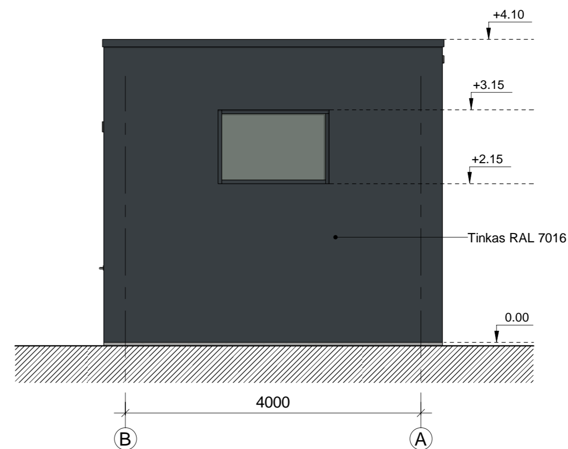
Fasadas B-A
