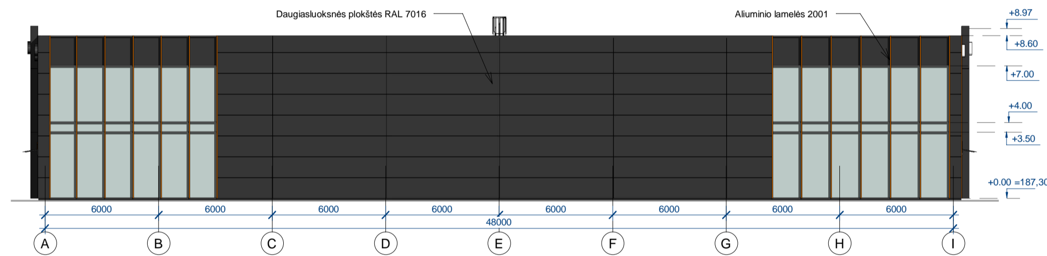
Fasadas A-I 1:200
