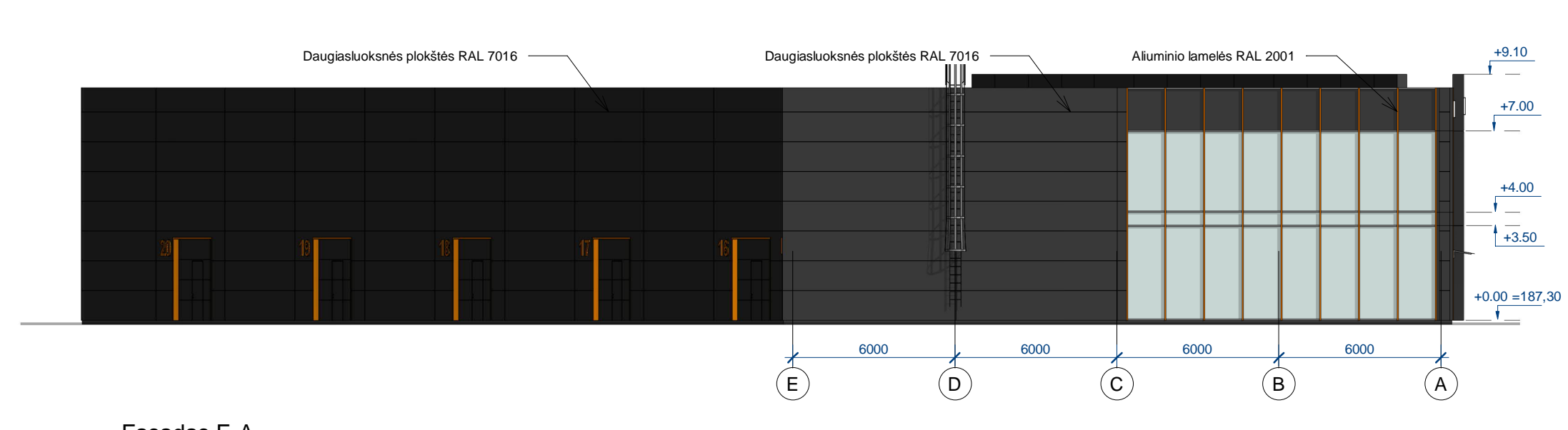
Fasadas E-A 1:200
