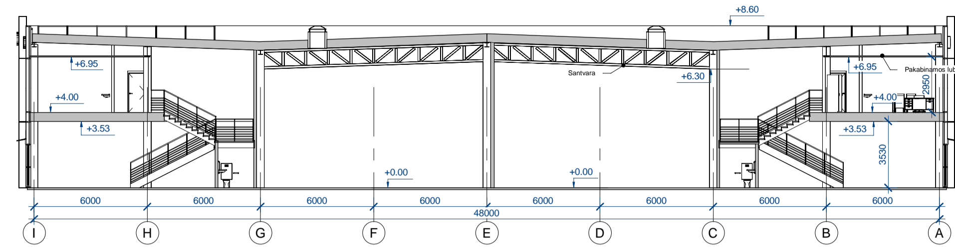
Pjūvis 1-1 1:200
