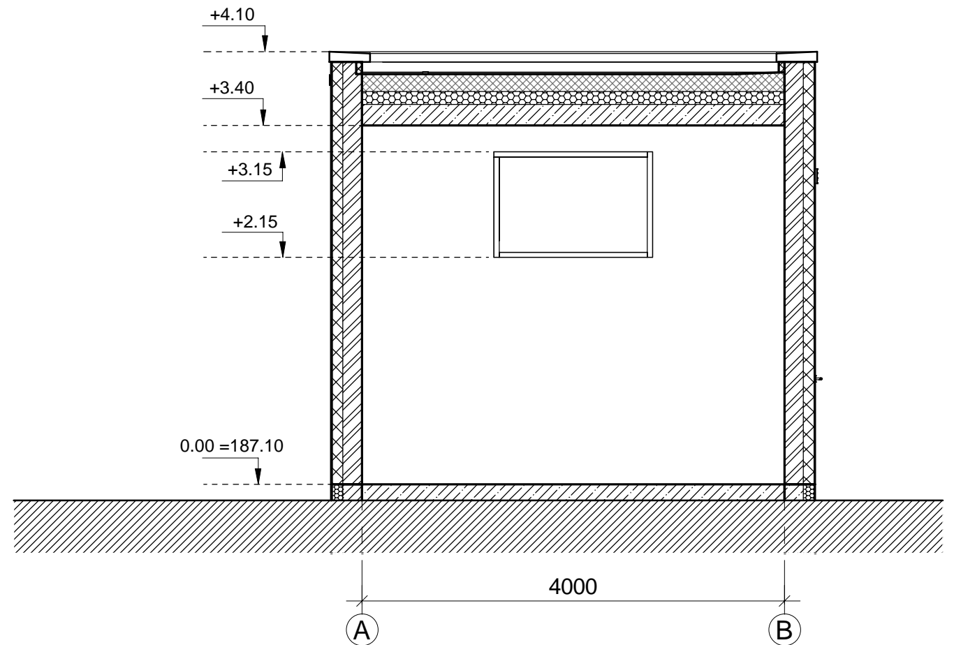
Pjūvis 1-1
