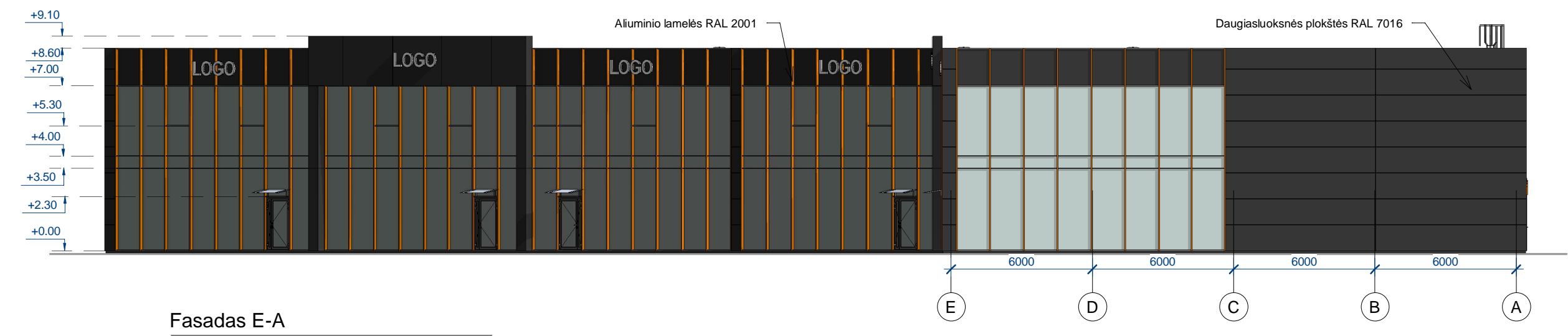
Fasadas E-A 1:200
