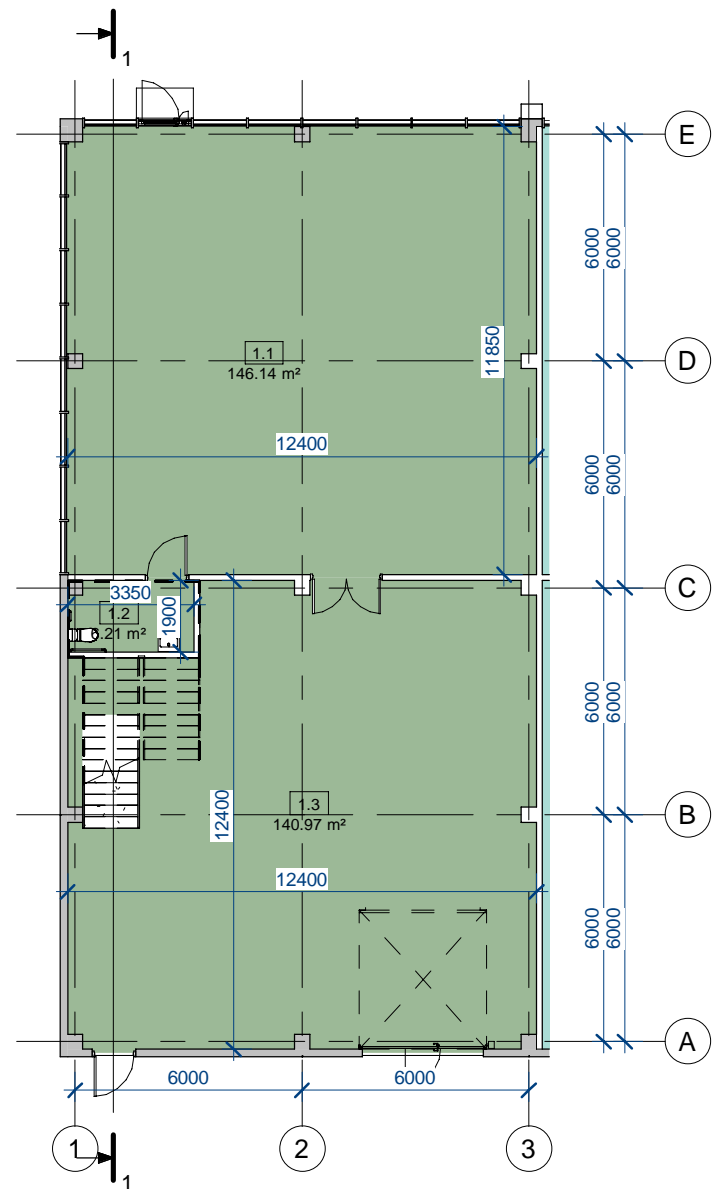
Pirmo aukšto plano ištrauka
