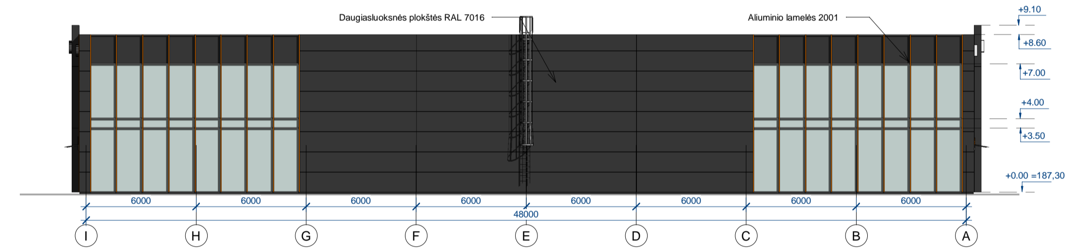
Fasadas I-A 1:200
