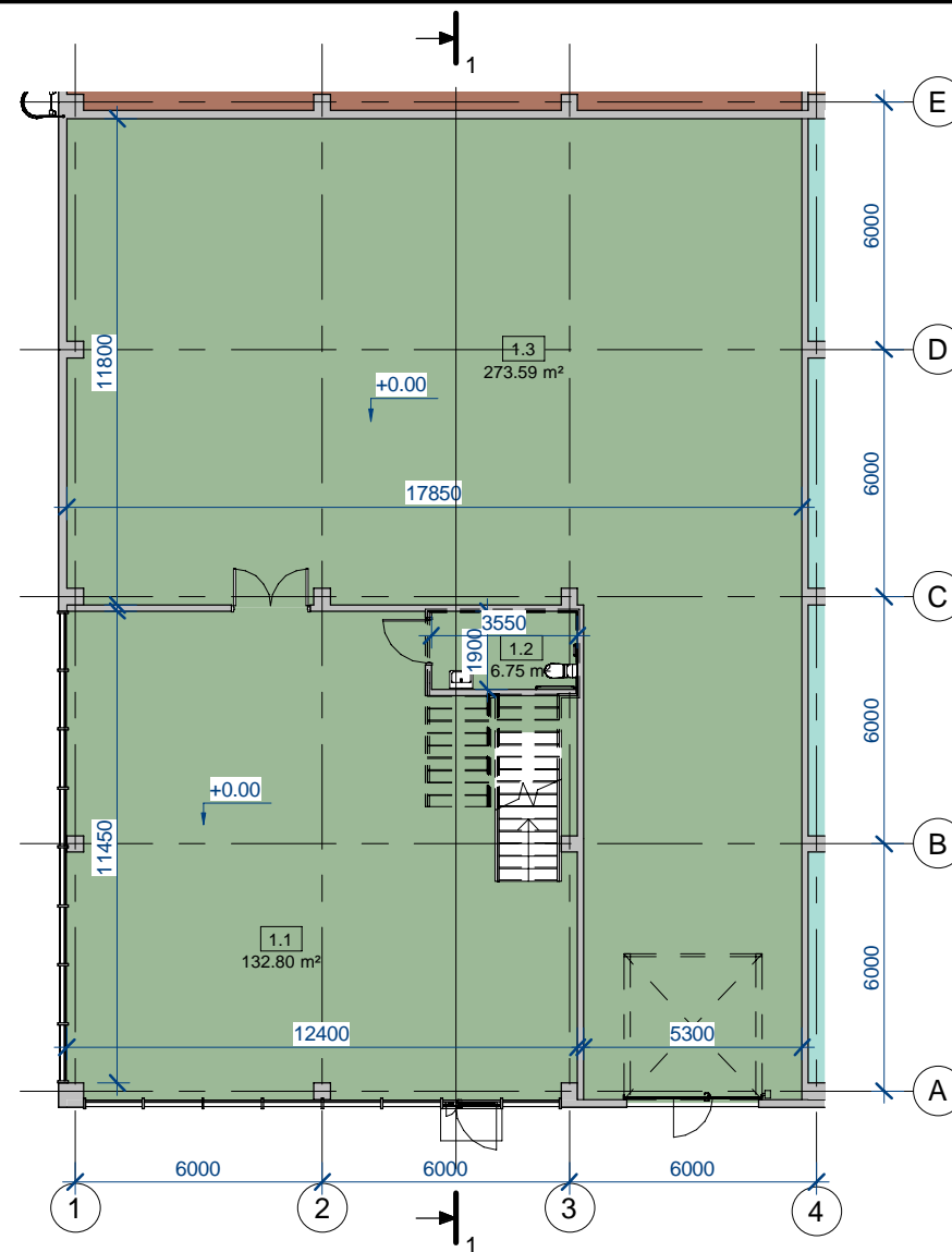
Pirmo aukšto plano ištrauka
