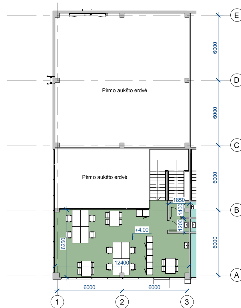
Antresolės plano ištrauka
