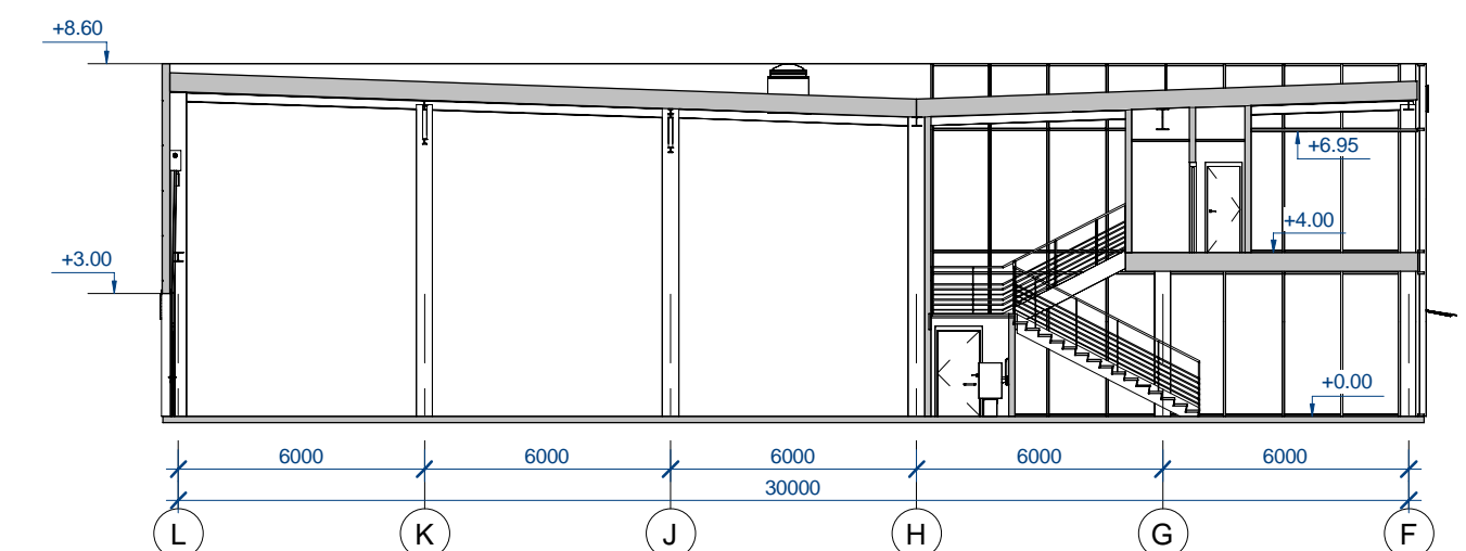
Pijvis 2-2 1:200
