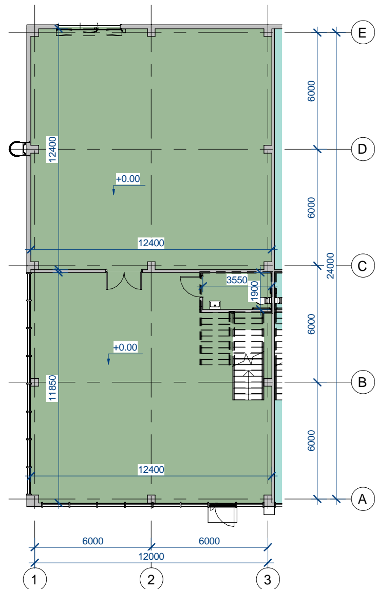
Pirmo aukšto plano ištrauka
