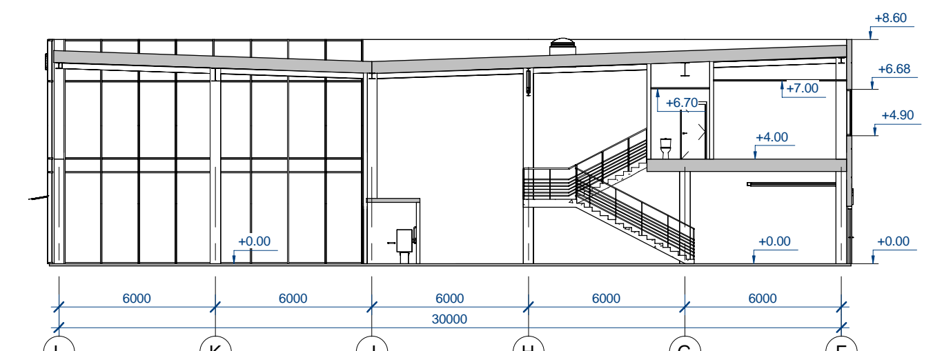
Pjūvis 2-2 1:200
