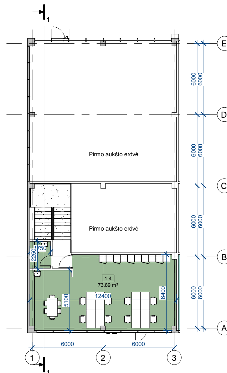
Antresolės plano ištrauka
