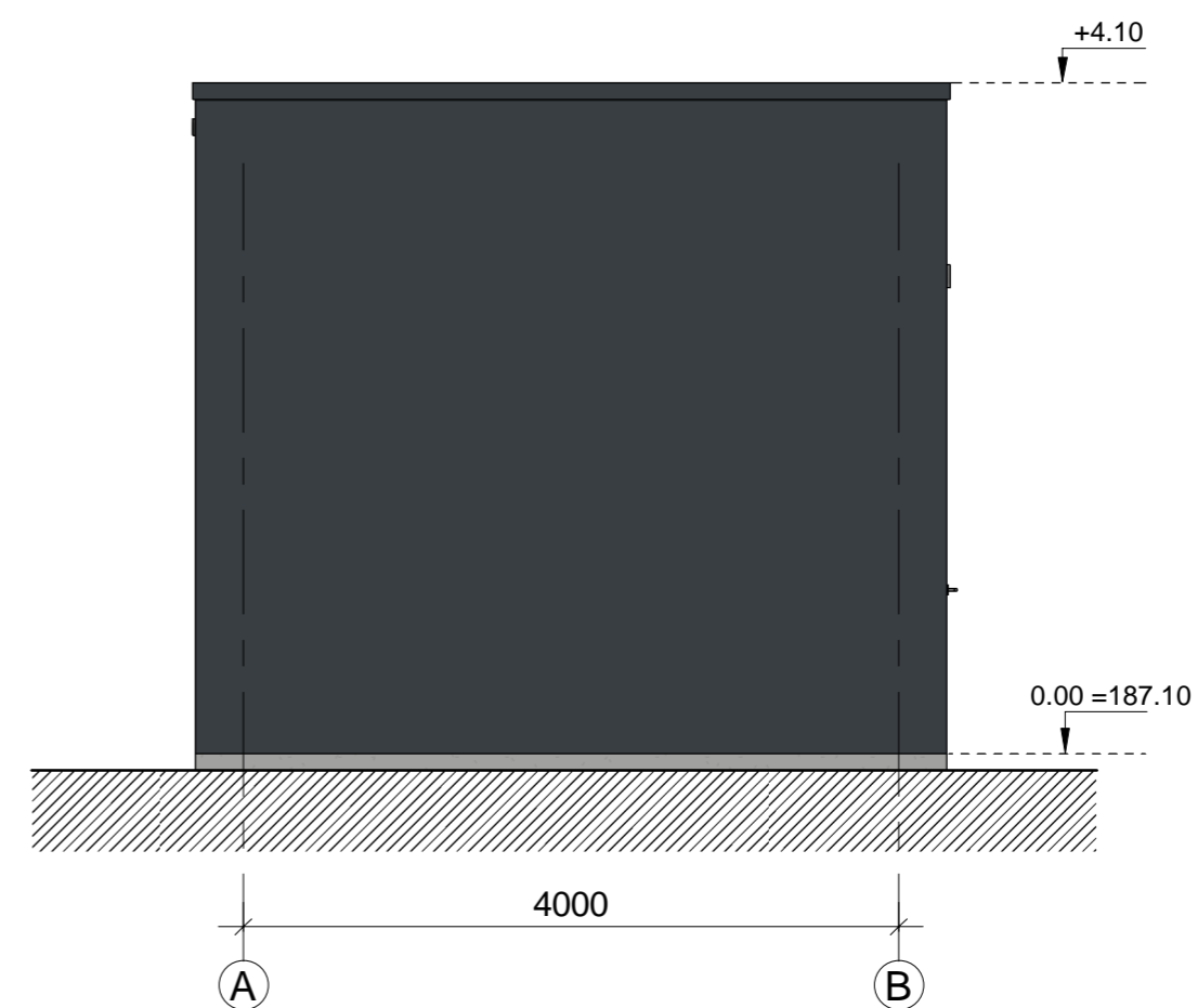
Fasadas A-B
