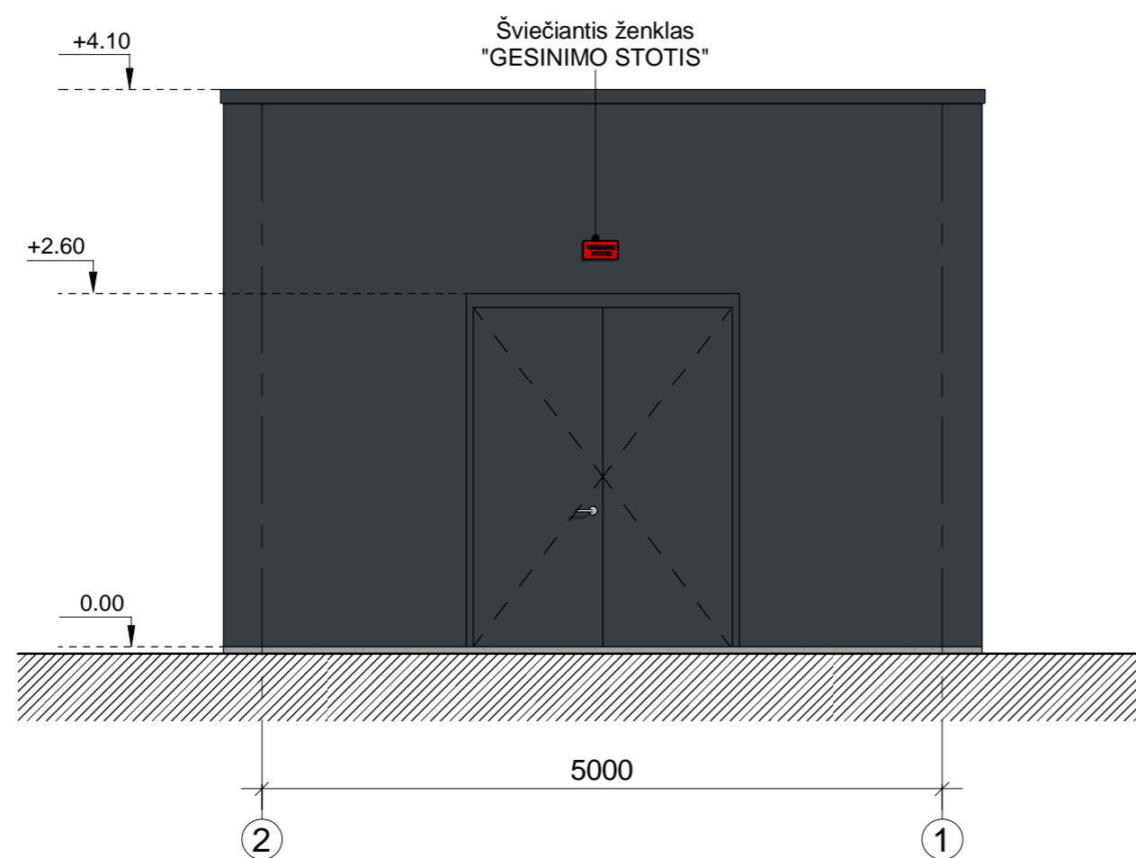
Fasadas 2-1
