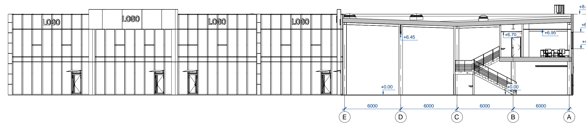
Pjūvis 1-1 1:200
